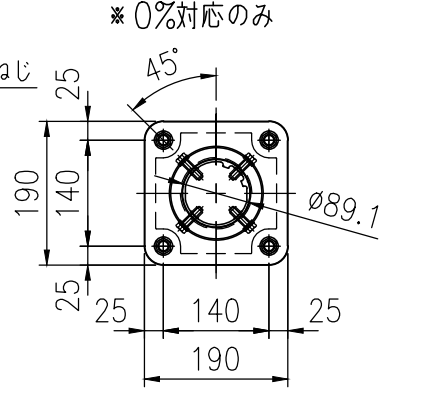
ベースプレート詳細図 (1/10)
