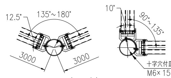
主要部材一覧 (S=1/5)
