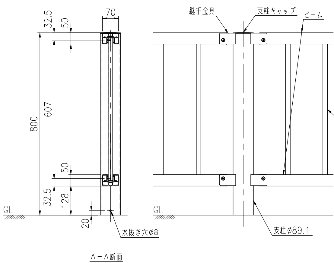
詳細図 (1/10)
