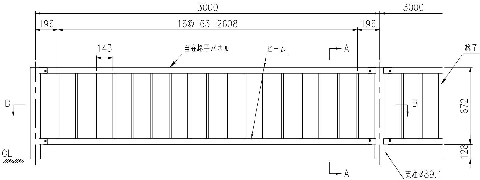
設置図 (1/20)
