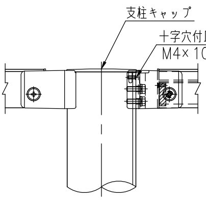
支柱キャップ納まり (1/5)
