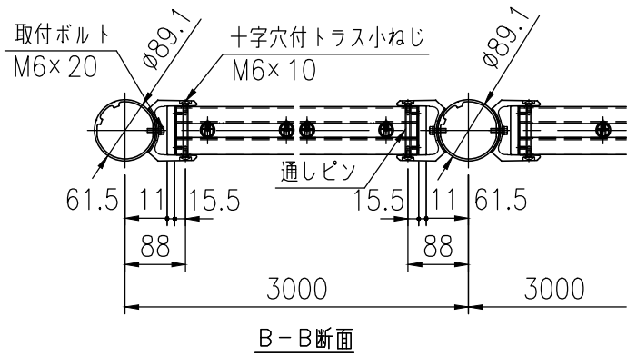
コーナー納まり (1/10)
