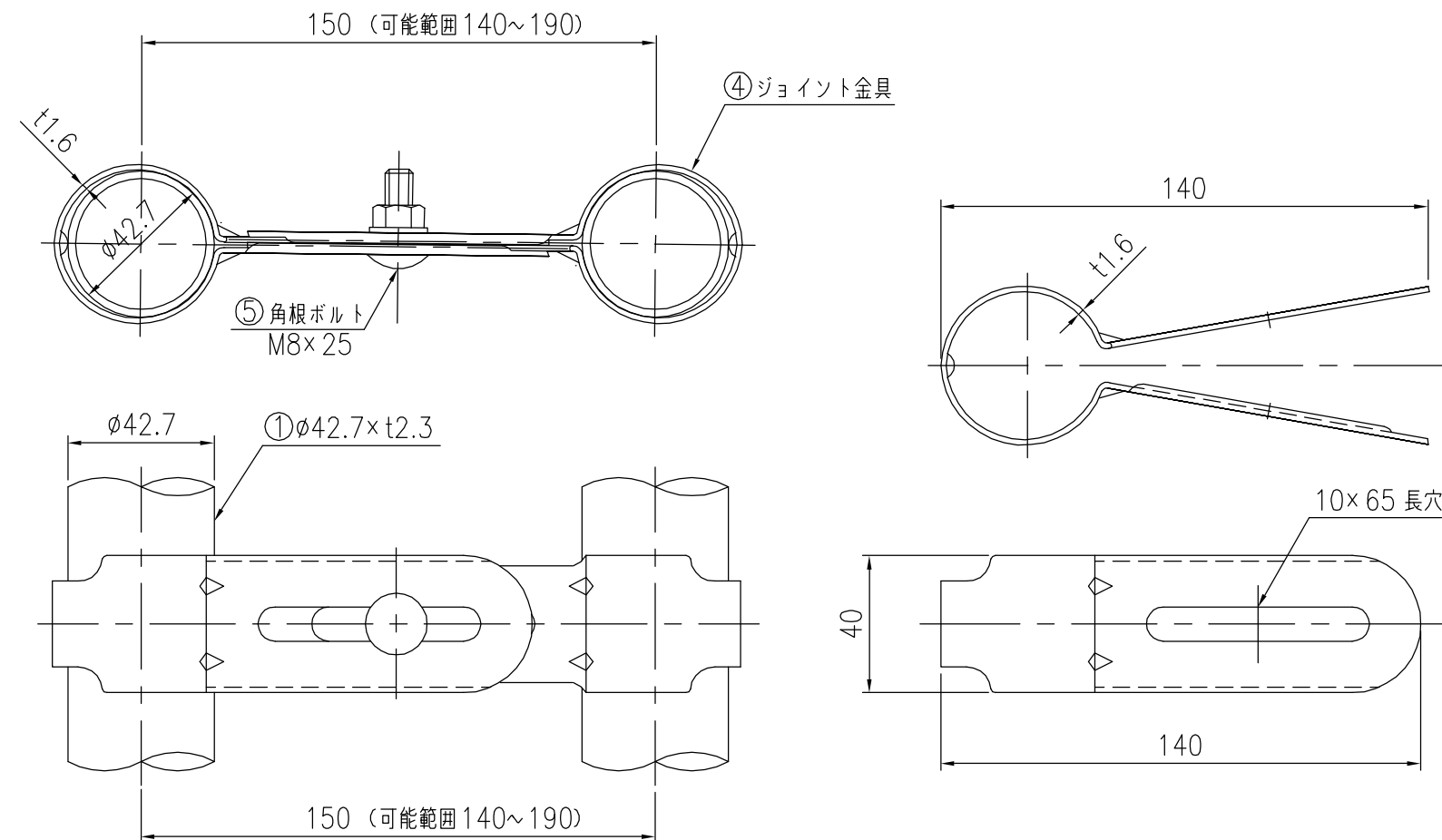
ジョイント金具詳細図 (1/2)
