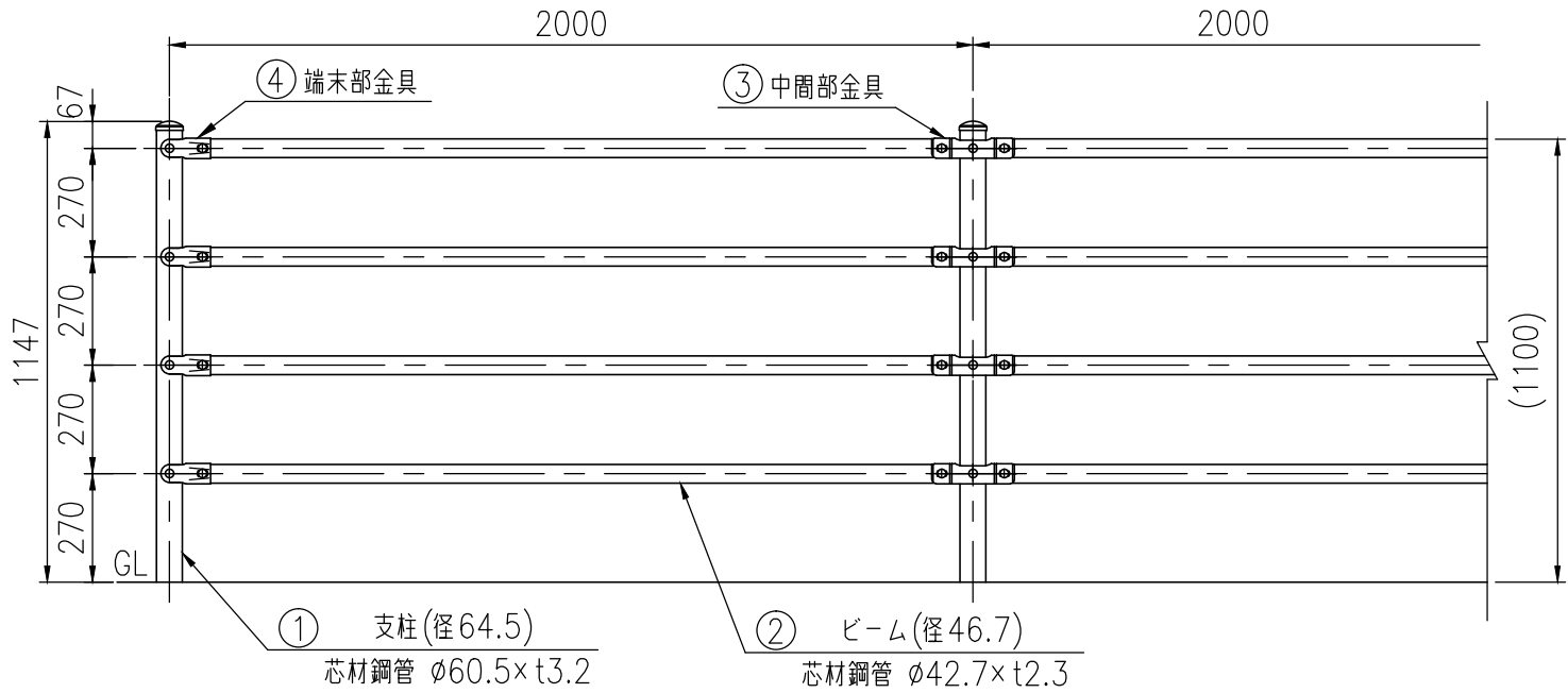
設置図 (1/20)
