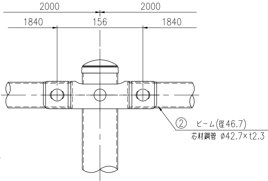
取付部詳細図 (1/4)
