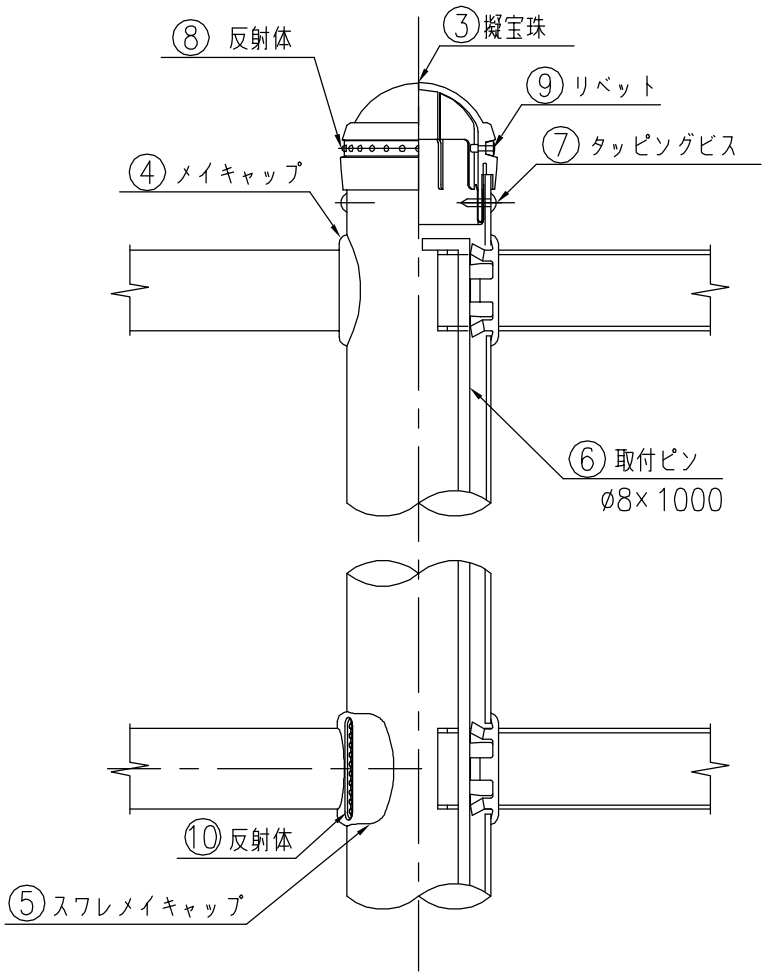
取付部詳細図 (1/4)
