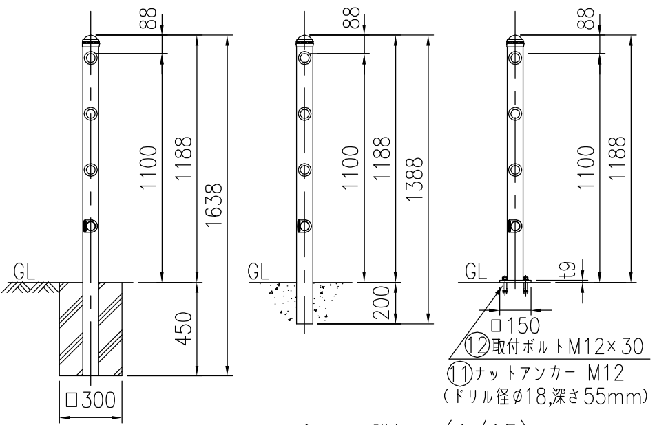
ベースプレート詳細図 (1/15)
