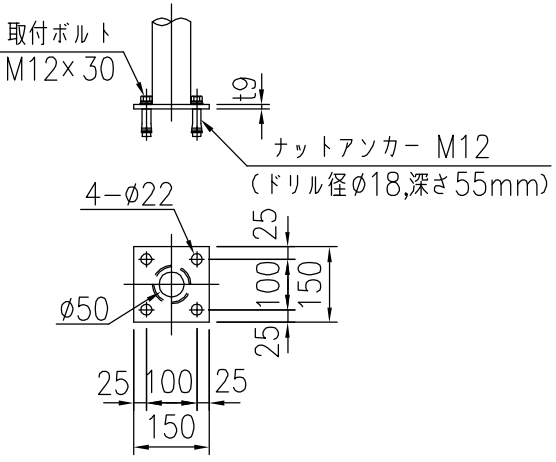
ベースプレート詳細図 (1/15)
