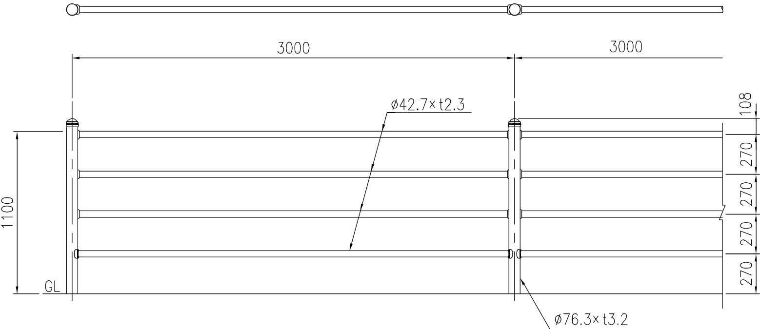
設置図 (1/25)
