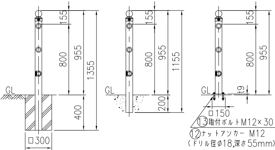
ベースプレート詳細図 (1/15)
