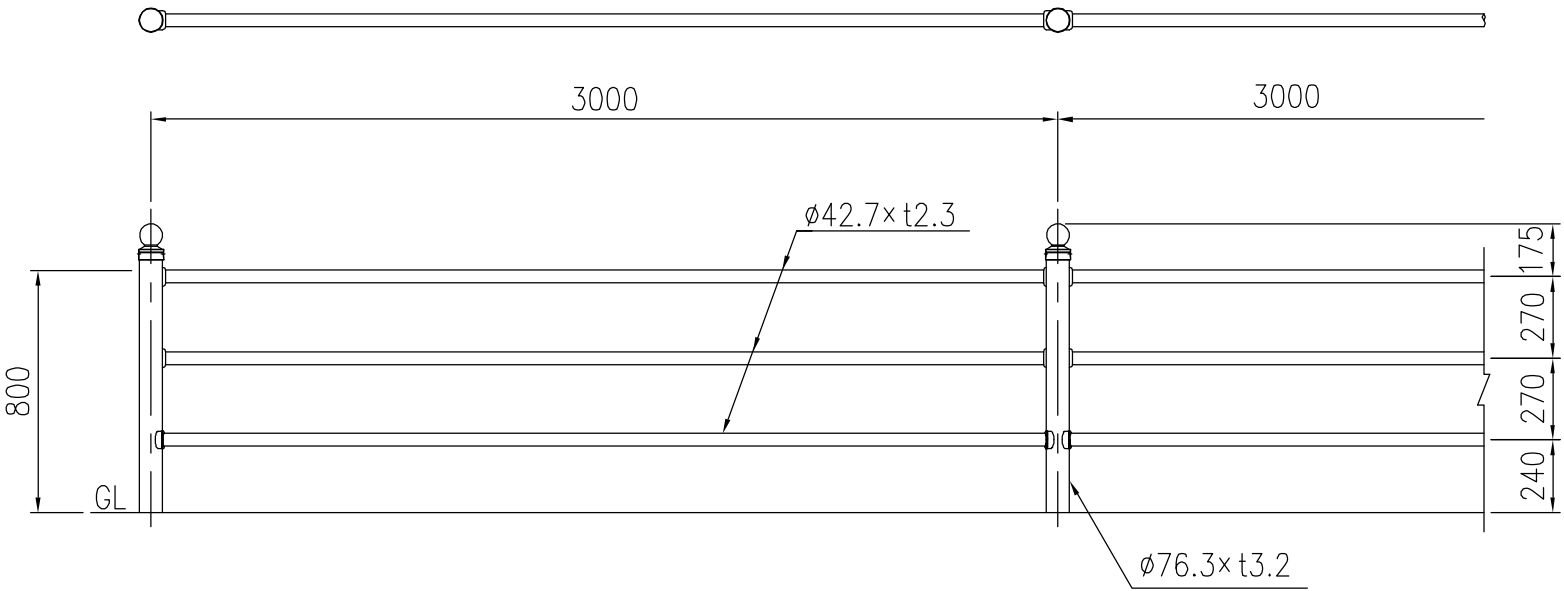
設置図 (1/25)
