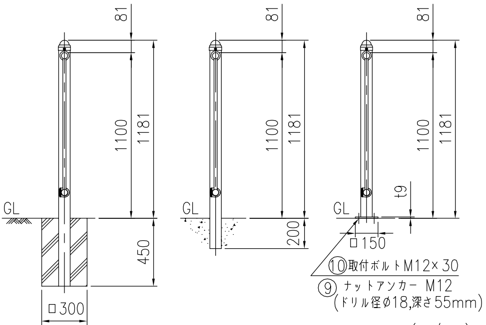
ベースプレート詳細図 (1/10)
