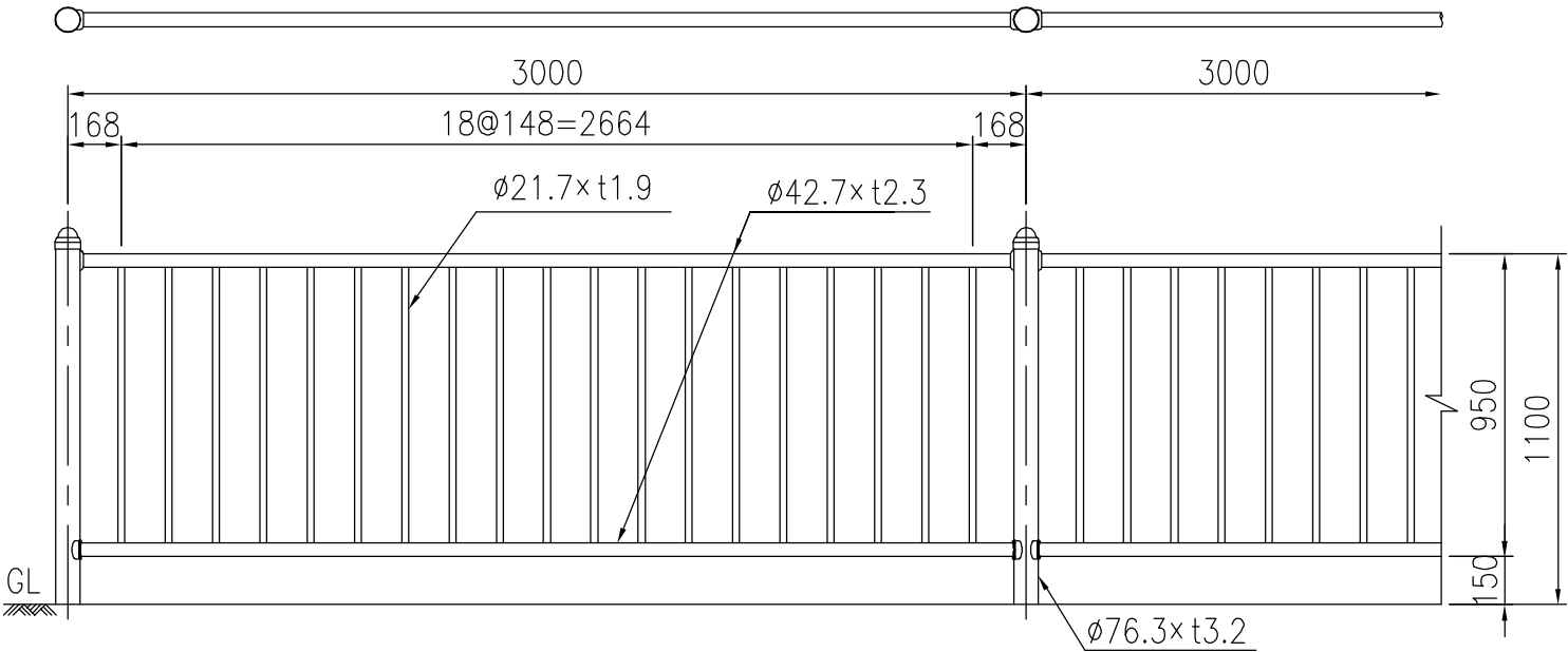
支柱図 (1/10)
