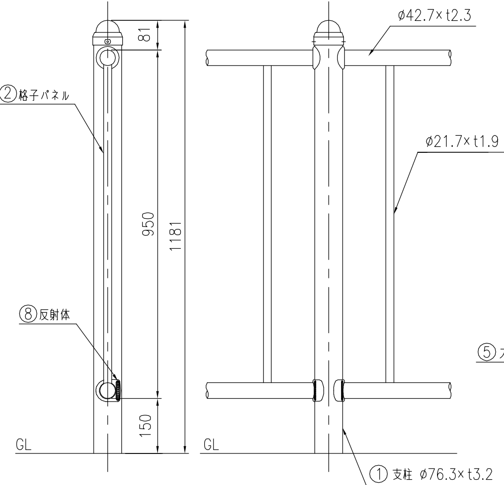
支柱図 (1/10)
