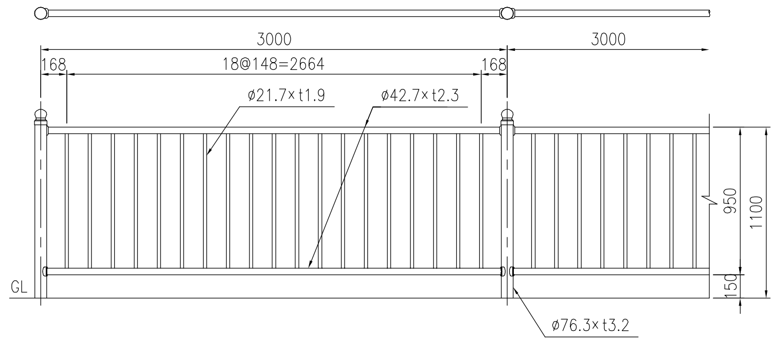
設置図 (1/25)
