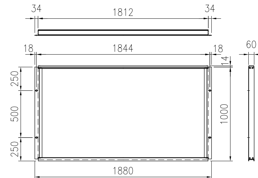
パネル (採光タイプ H1m) 詳細図 (1/25)
