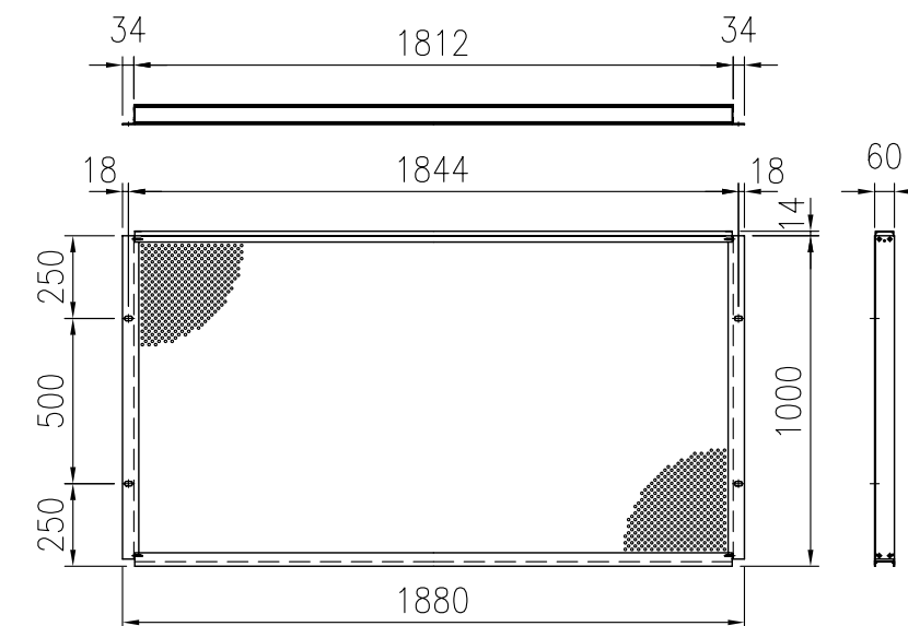
パネル (吸音タイプ H1m) 詳細図 (1/25)
