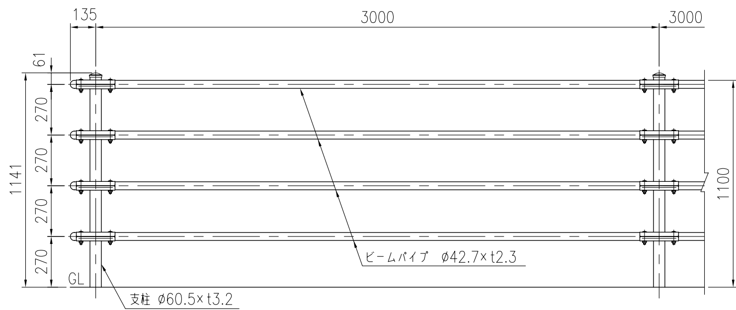
設置図 (1/20)
