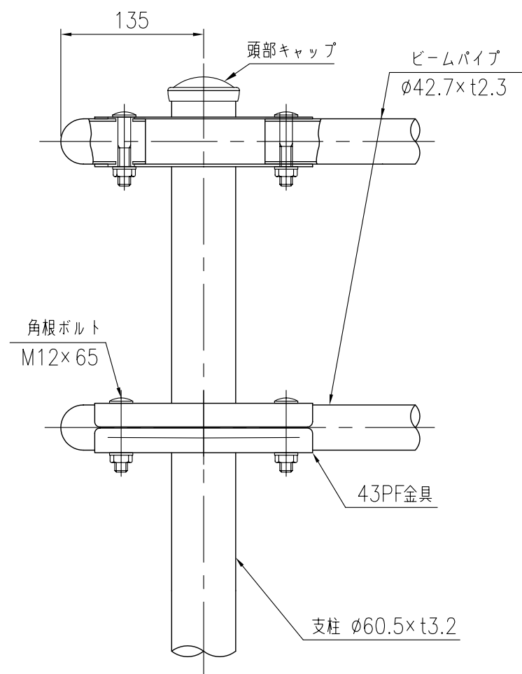
支柱図 (1/5)
