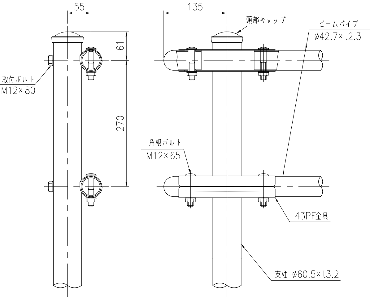
支柱図 (1/5)
