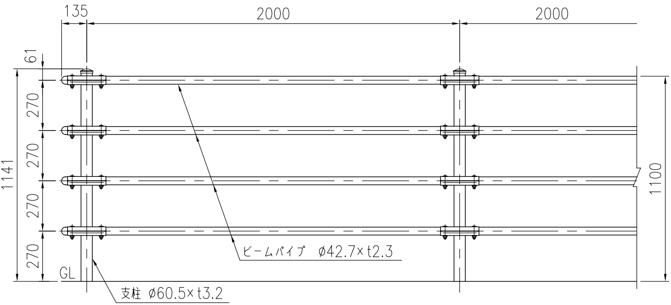
設置図 (1/20)
