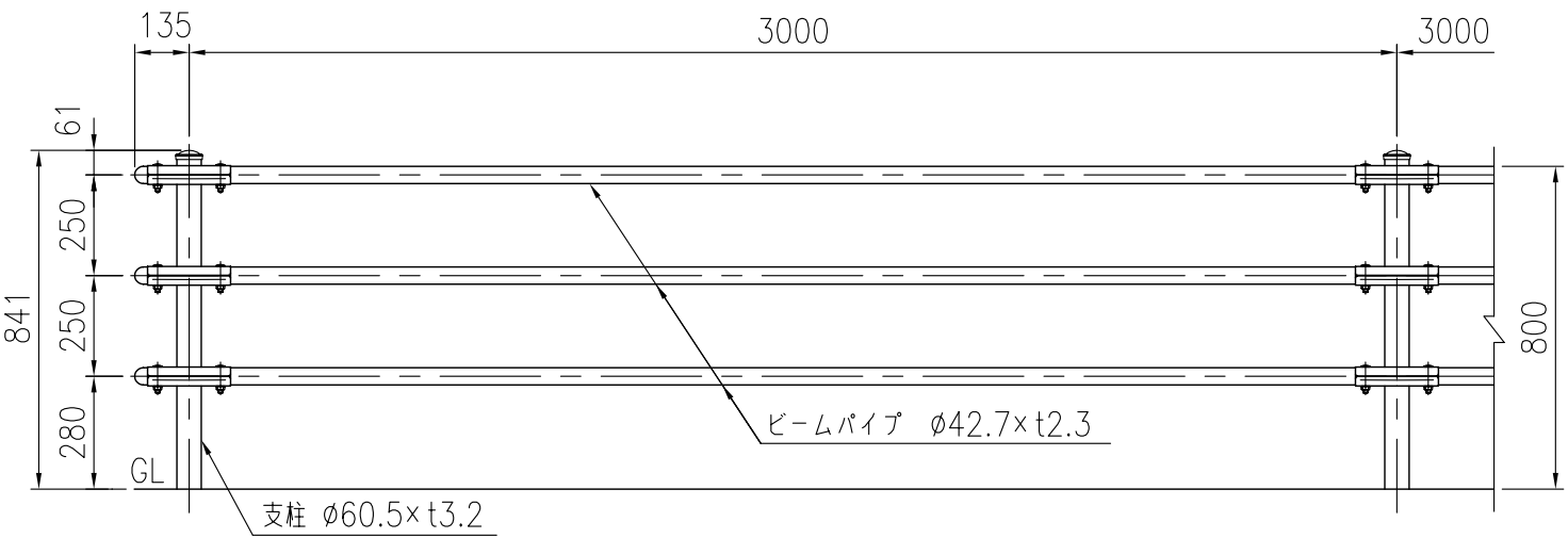
支柱図 (1/5)
