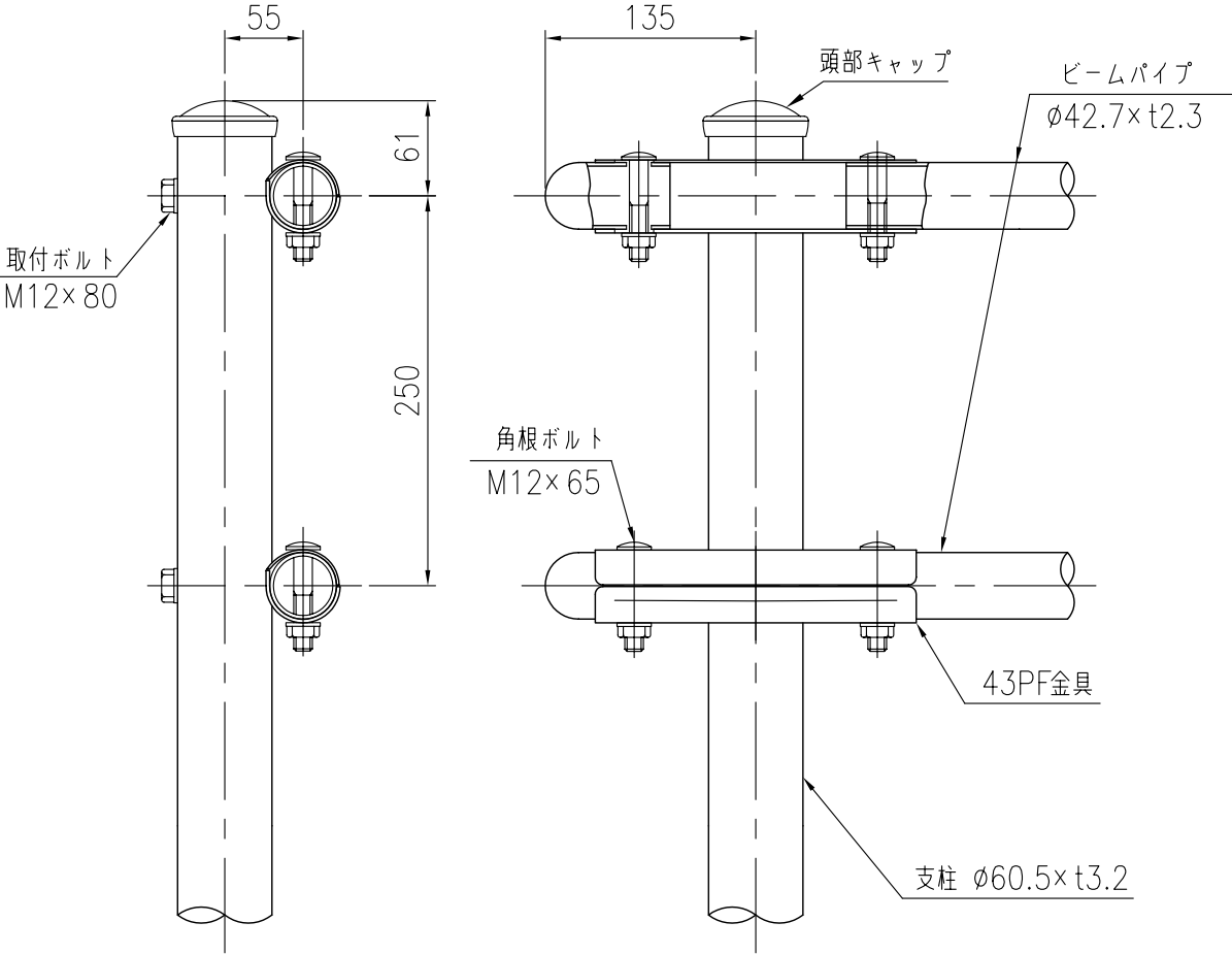
支柱図 (1/5)
