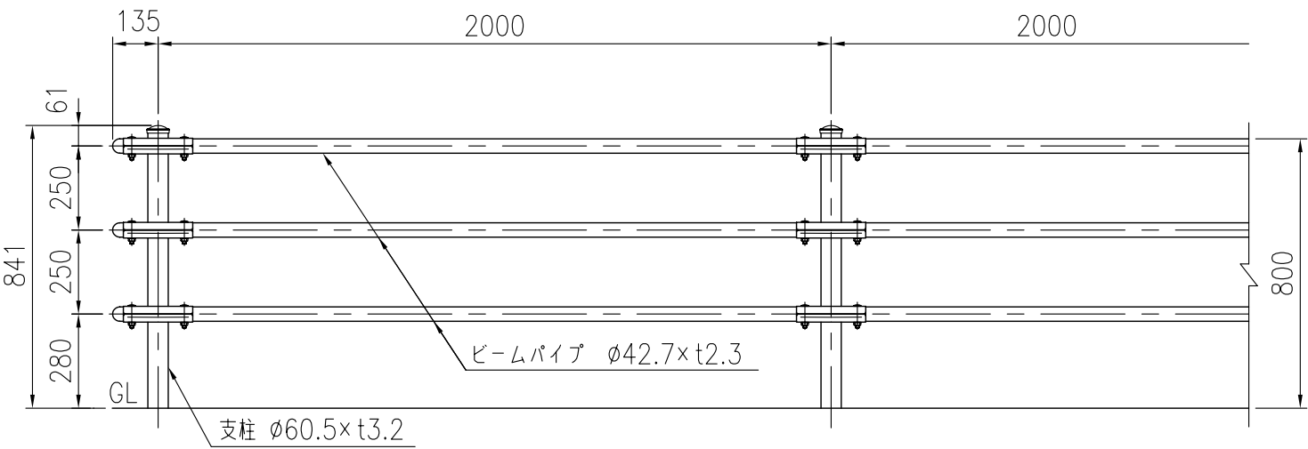
支柱図 (1/5)
