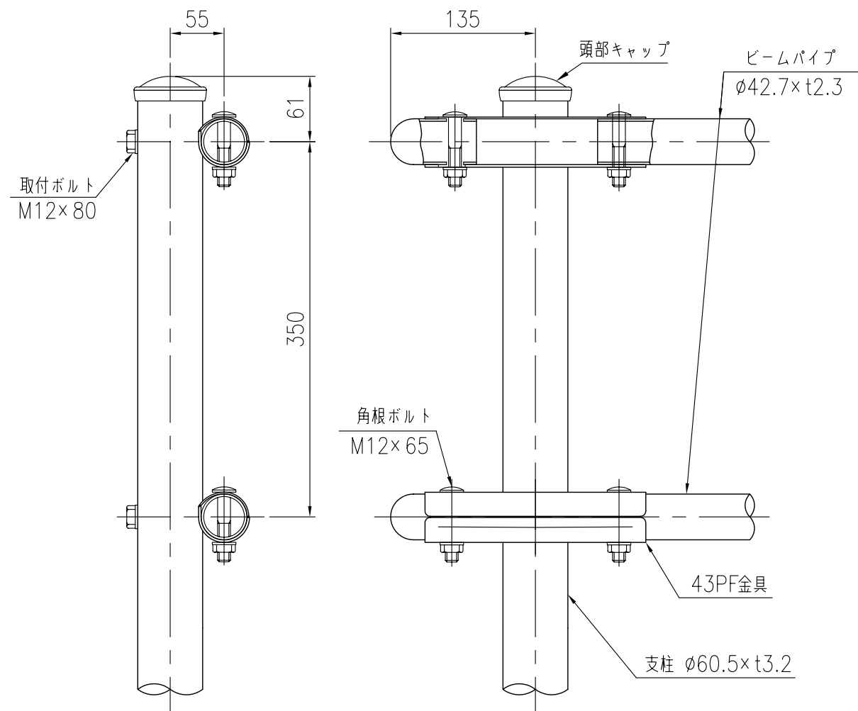
支柱図 (1/5)
