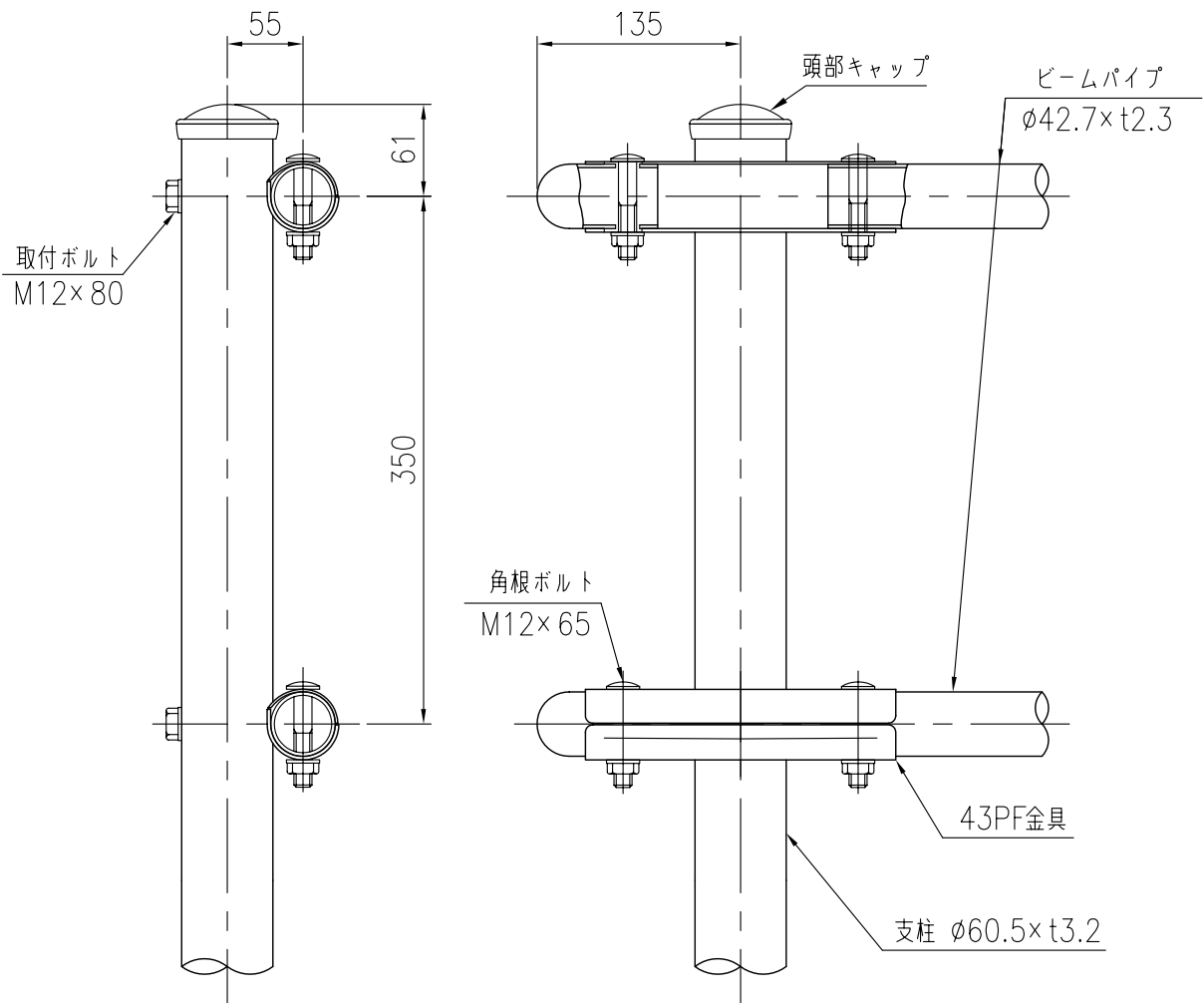
支柱図 (1/5)
