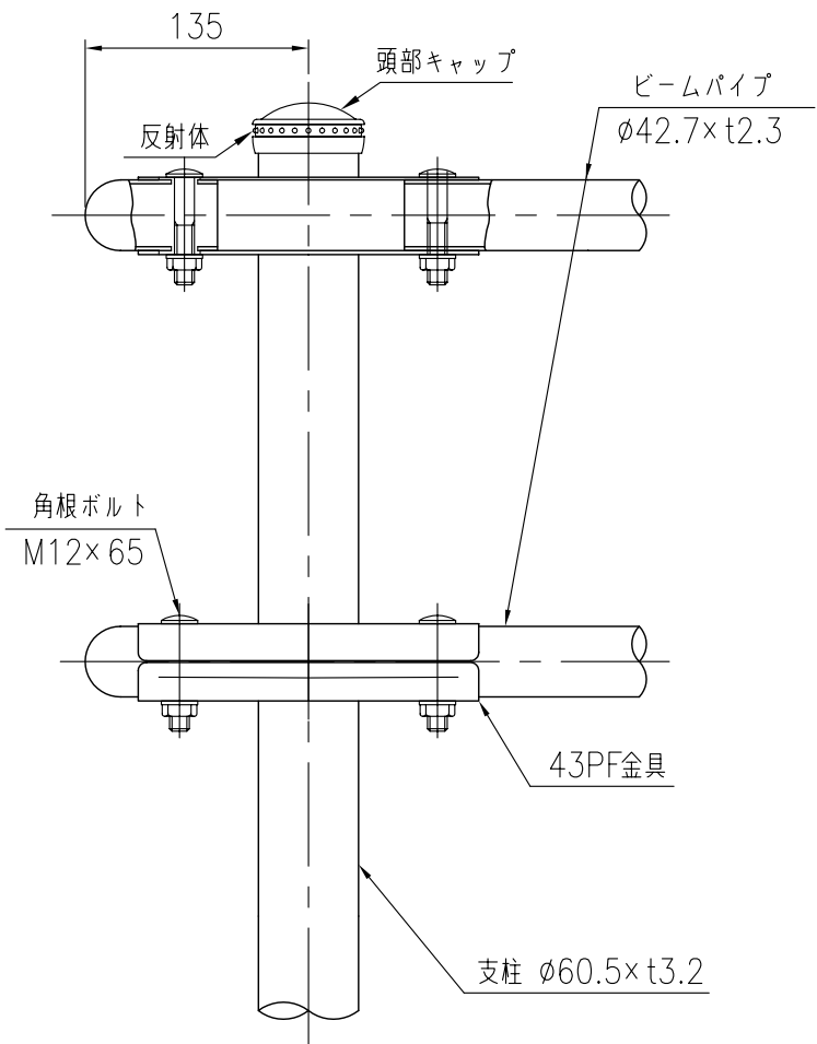
支柱図 (1/5)
