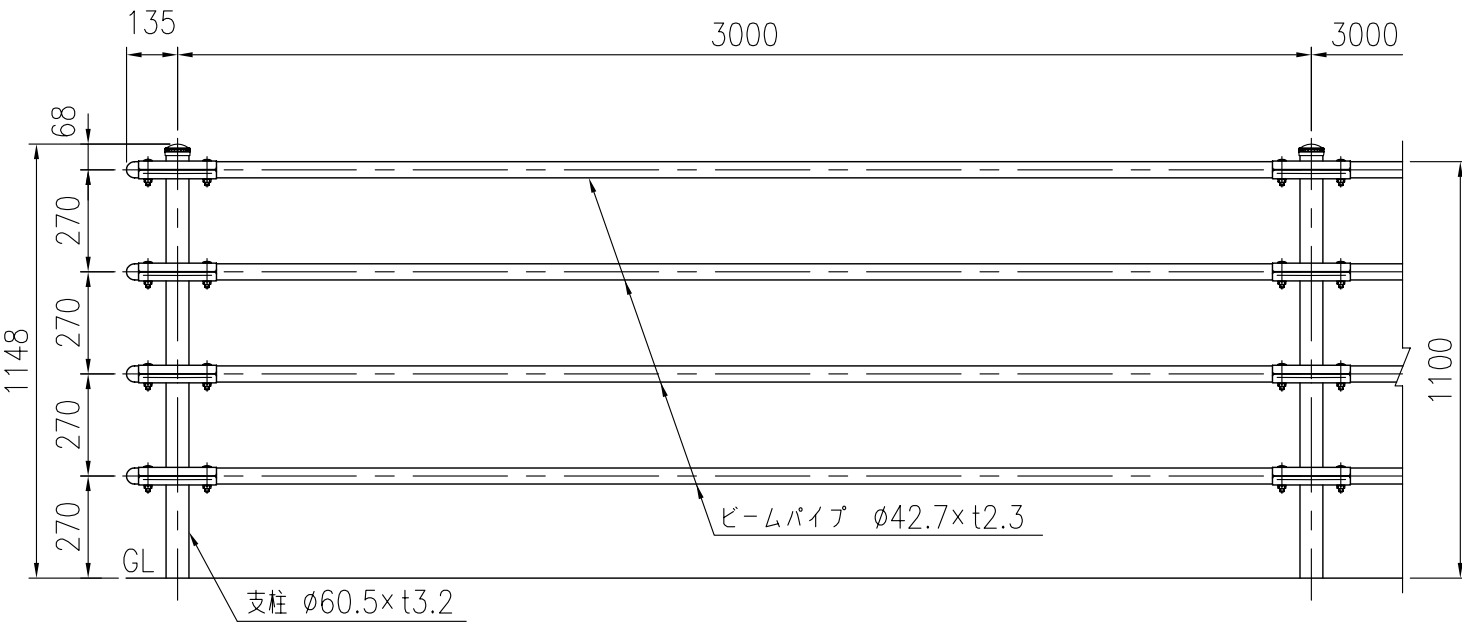
設置図 (1/20)
