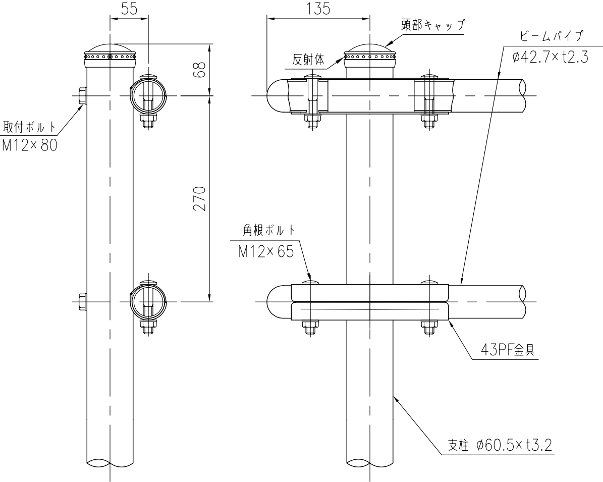
支柱図 (1/5)
