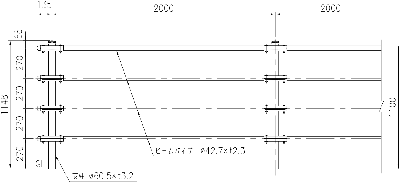
設置図 (1/20)
