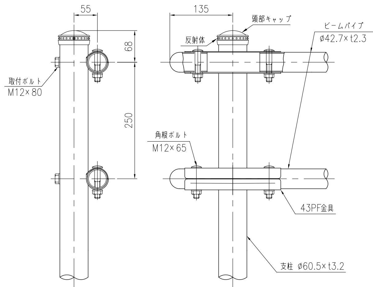
支柱図 (1/5)
