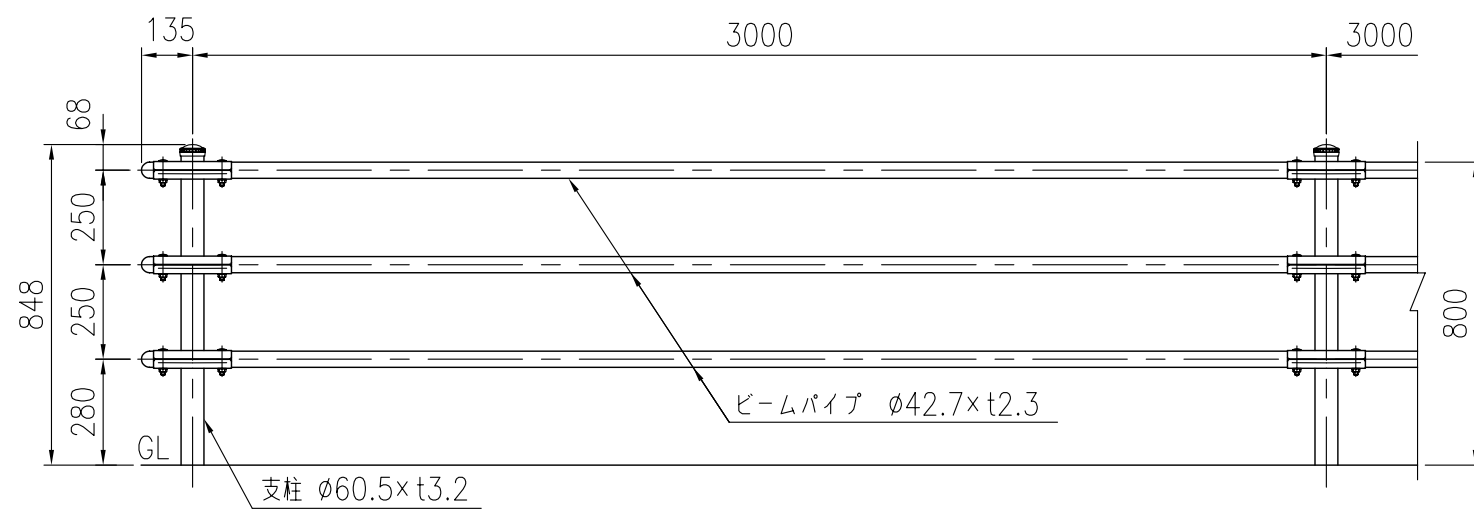
設置図 (1/20)
