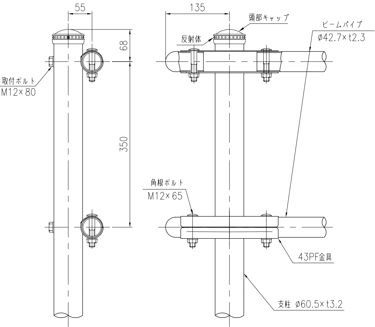
支柱図 (1/5)
