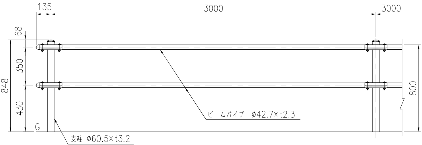
設置図 (1/20)
