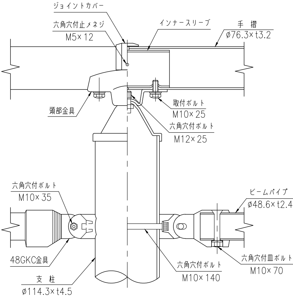
取付部詳細図 (1/4)
