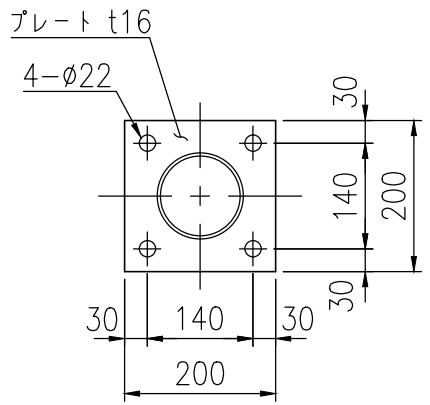
ベースプレート詳細図 (1/10)
