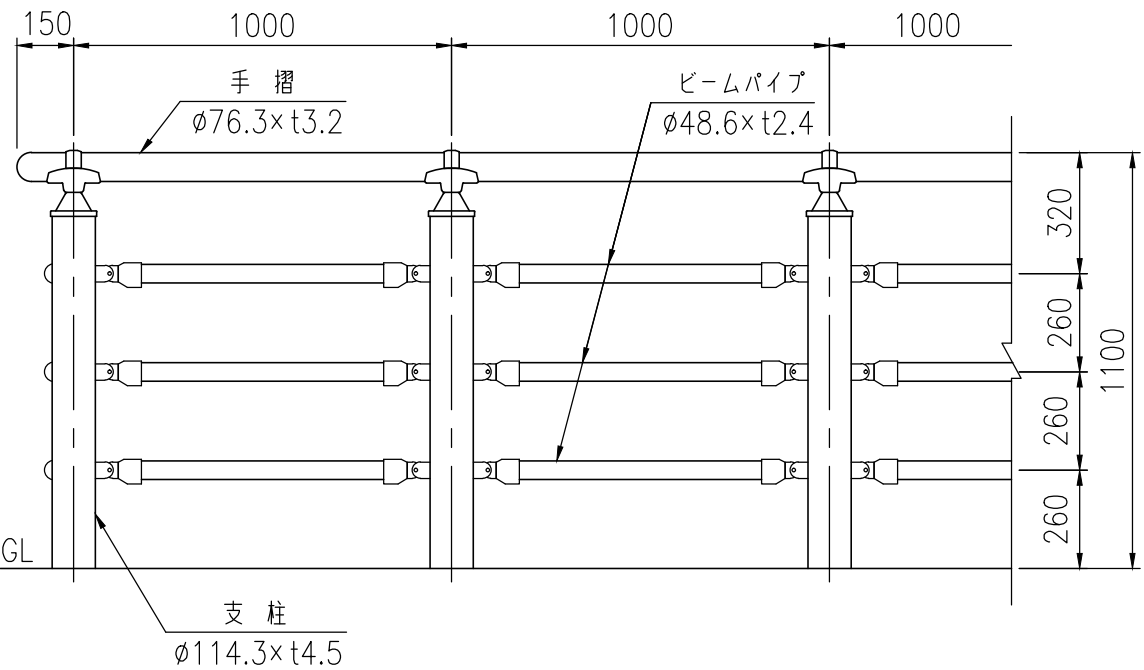
取付部詳細図 (1/4)
