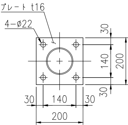
ベースプレート詳細図 (1/10)
