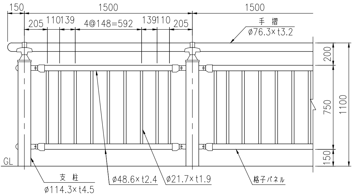
設置図 (1/20)
