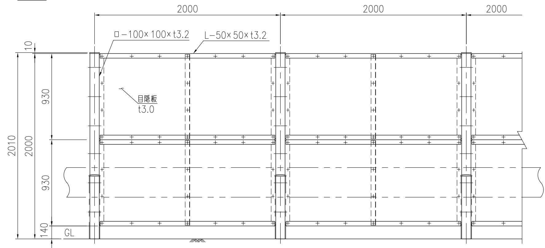
設置図 (1/25)
