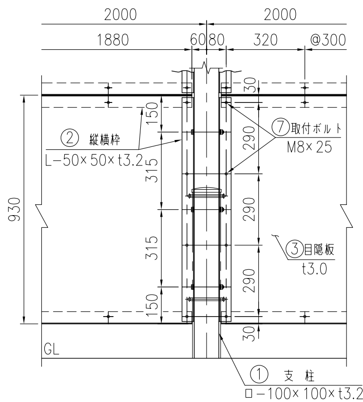
裏面図 (1/15)
