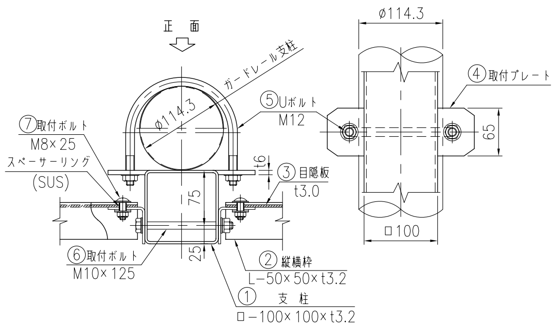
取付部詳細図 (1/5)
