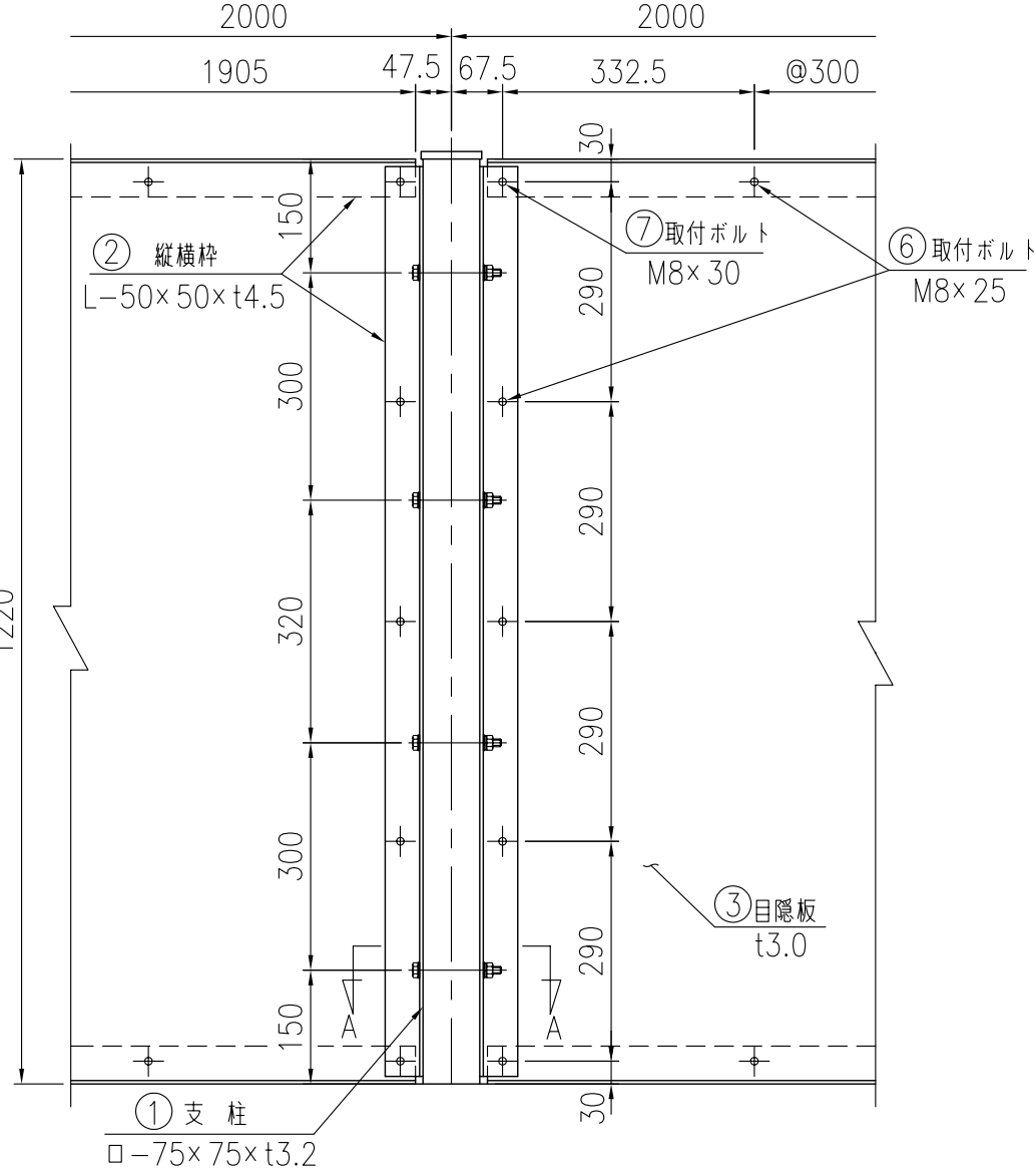
裏面図 (1/10)
