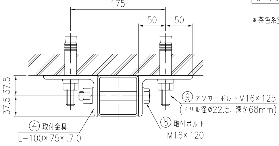
(B-B 断面図)
