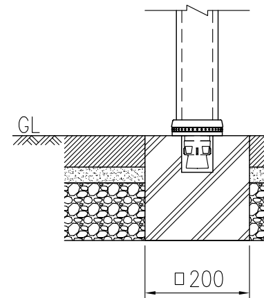
アンカー+コンクリート基礎
