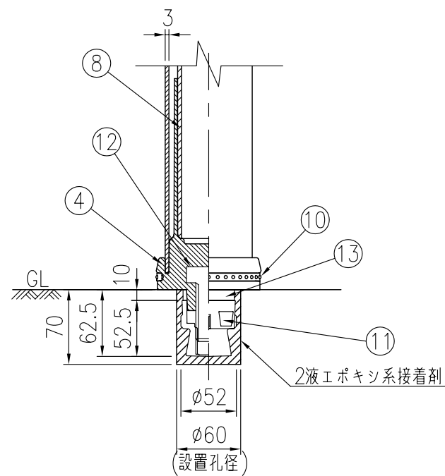
ベース部(設置図) S=1/5
