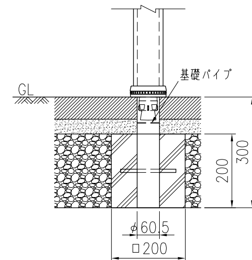
アンカー+基礎パイプ
