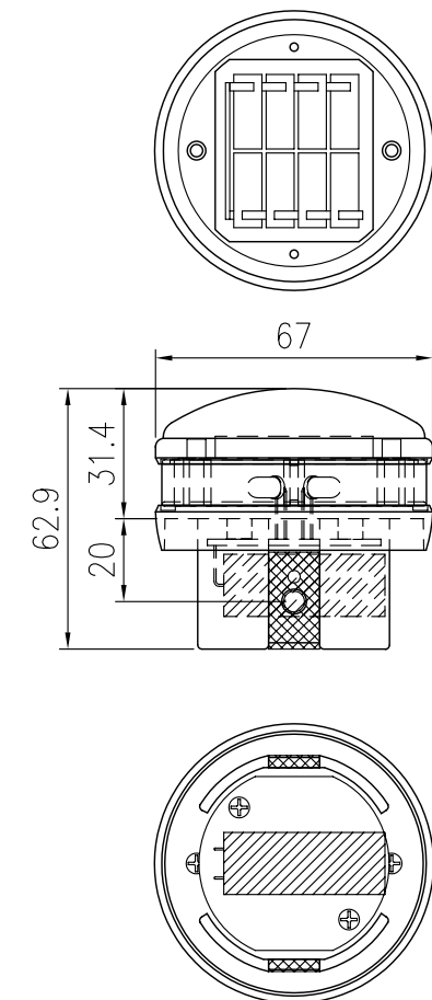
SLキャップ80 S=1/2
