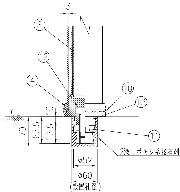
姿図 S=1/10
