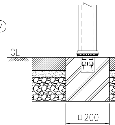
アンカー+コンクリート基礎
