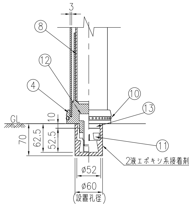
ベース部(設置図) S=1/5
