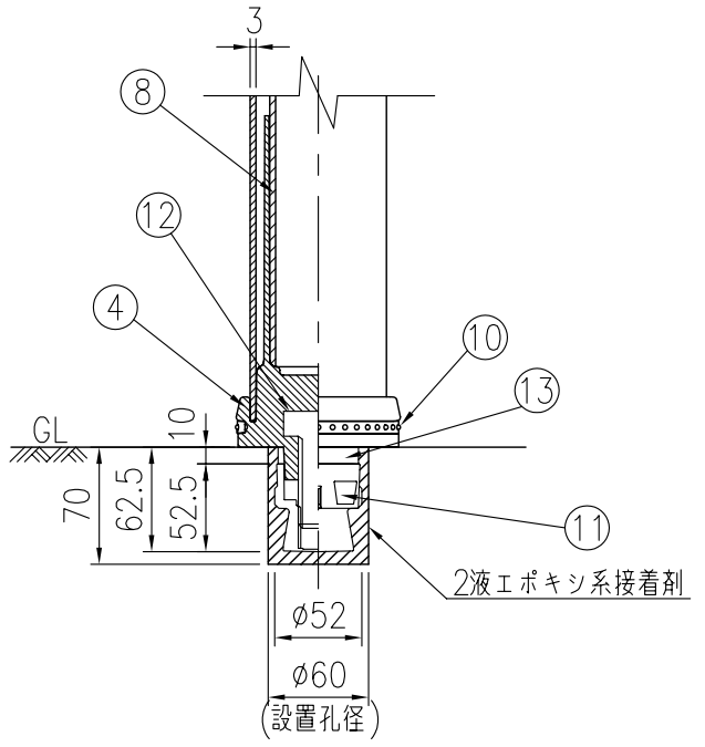
ベース部(設置図) S=1/5
