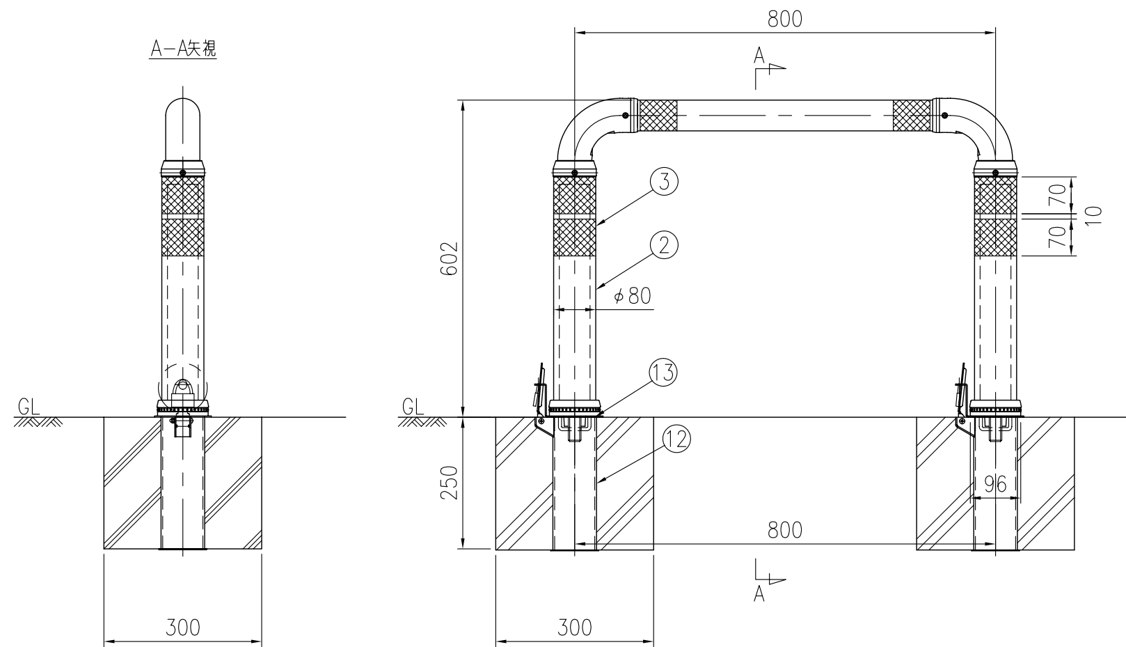
姿図 S=1/10
