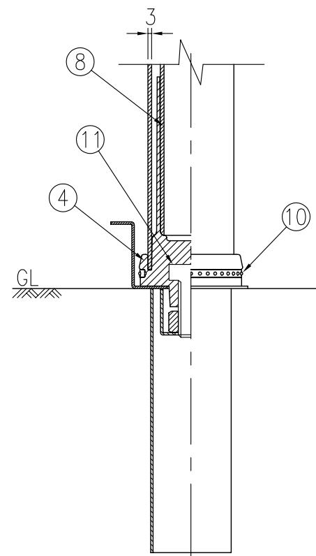
ベース部(設置図) S=1/5
