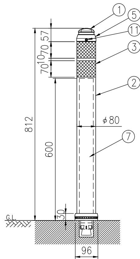
姿図 S=1/10
