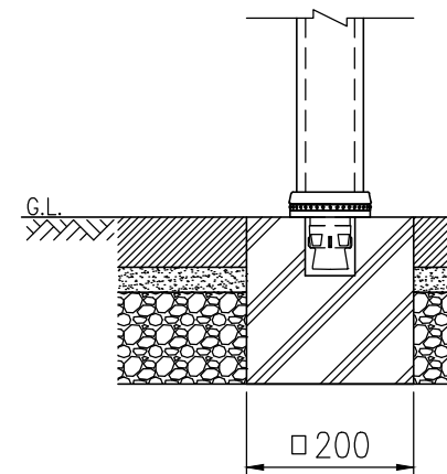
アンカー+コンクリート基礎
