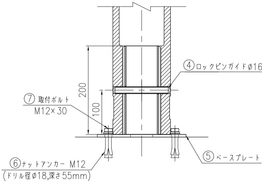
下部詳細断面図
