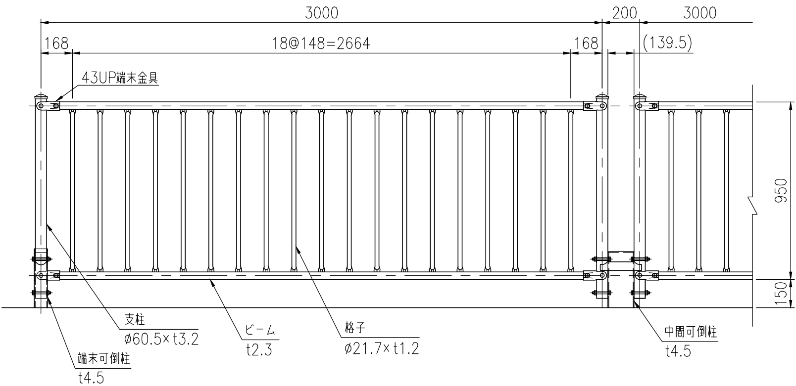
設置図 (1/20)
