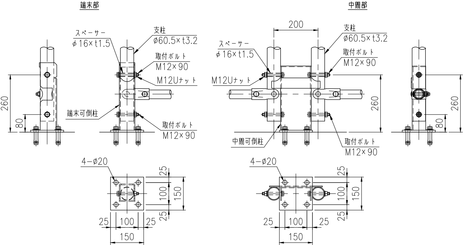
柱固定部詳細図 (1/10) (BPL式)
