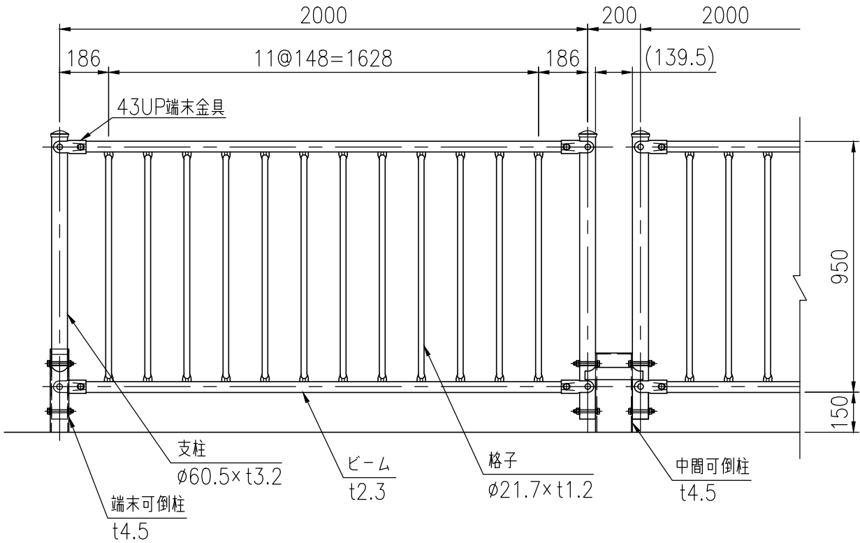
設置図 (1/20)
