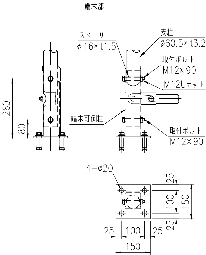
柱固定部詳細図 (1/10) (BPL式)
