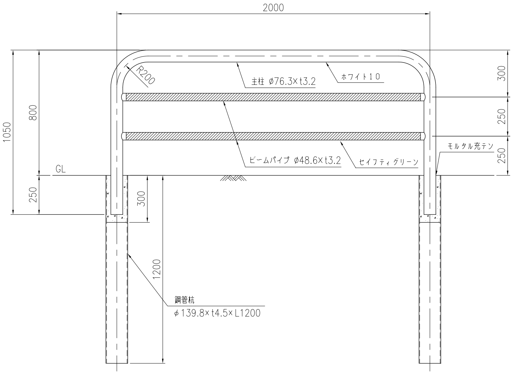
設置図
