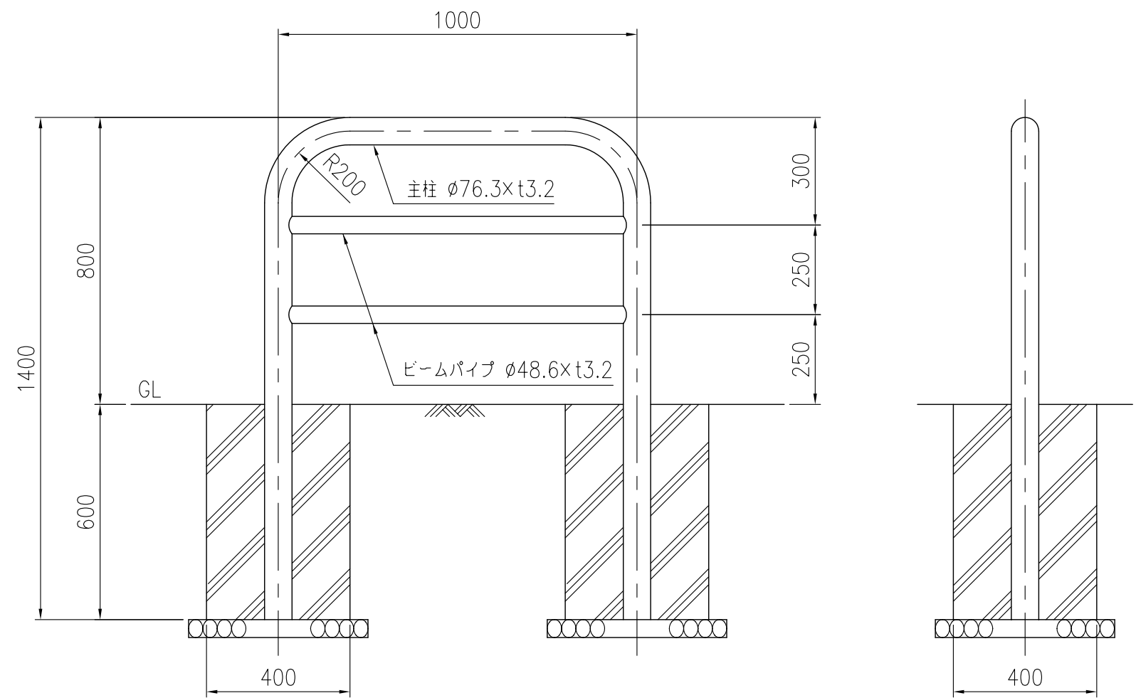
設置図
