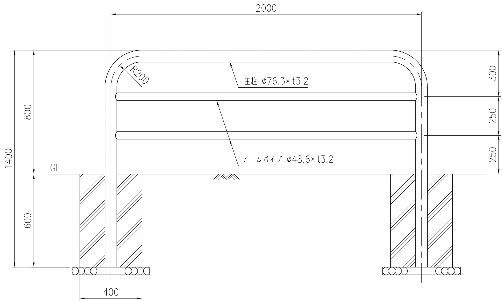
設置図
