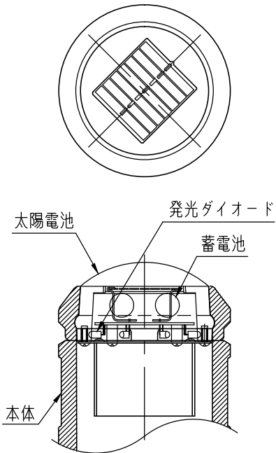
自発光頭部詳細図(1/4)
