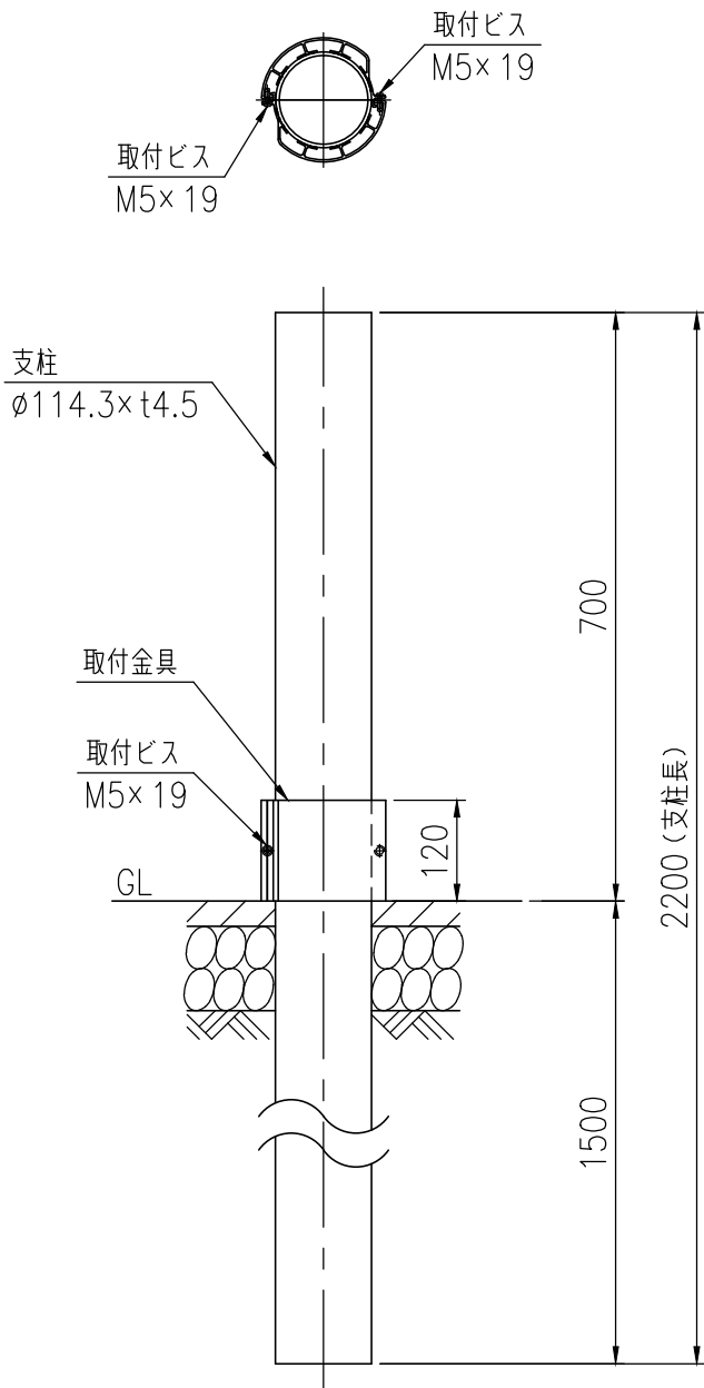
支柱設置図(1/10)
