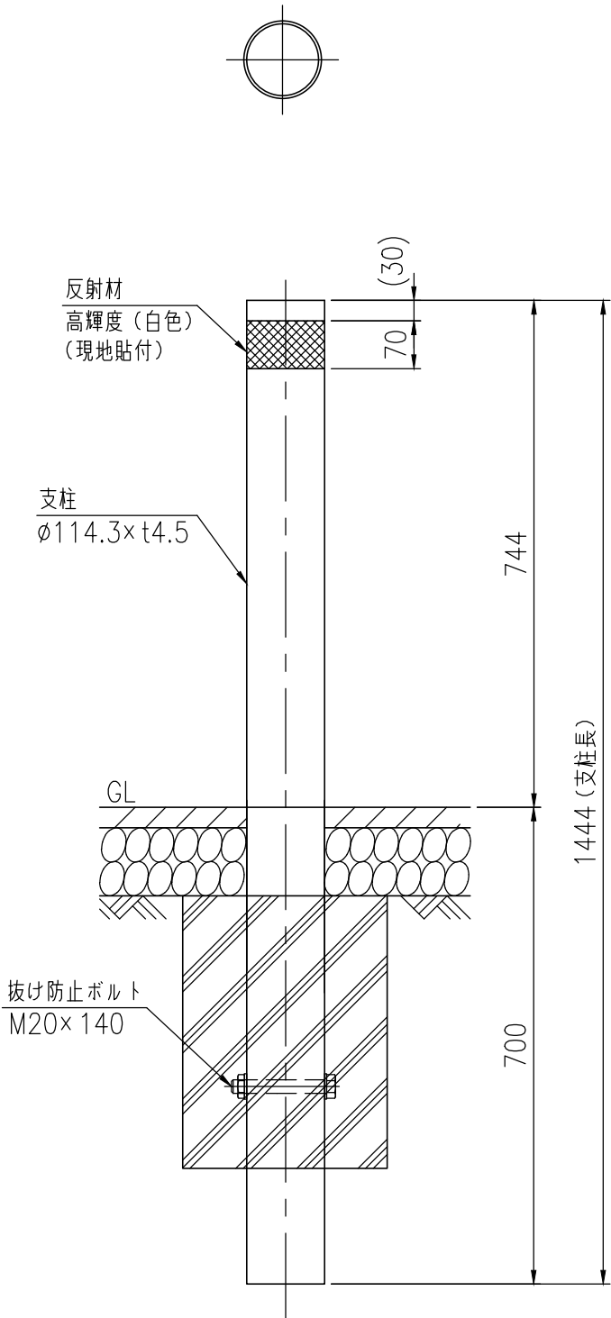
支柱設置図(1/10)
