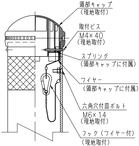
頭部キャップ取付詳細図(1/4)
