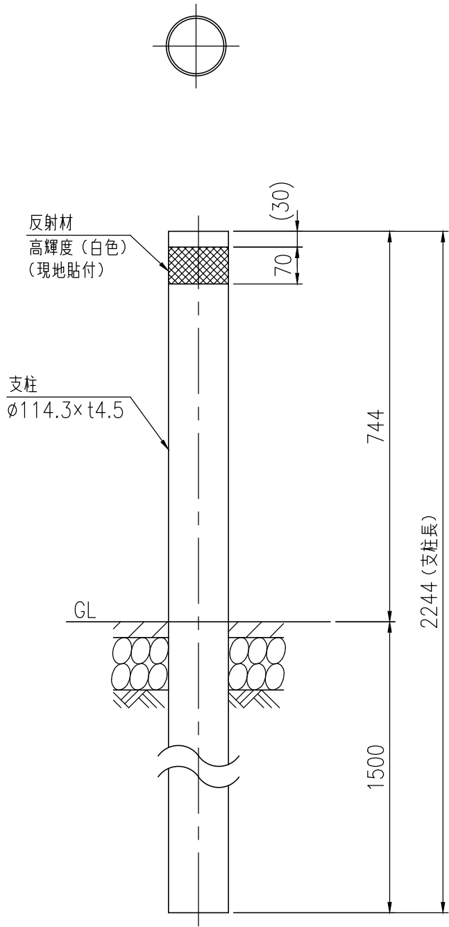
支柱設置図(1/10)
