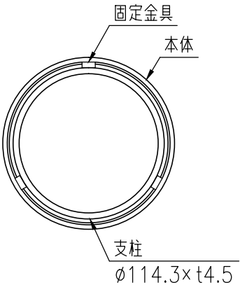
A-A 断面図 (1/4)
