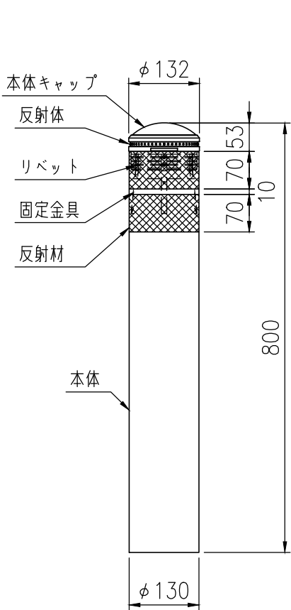
本体姿図 (1/10)
