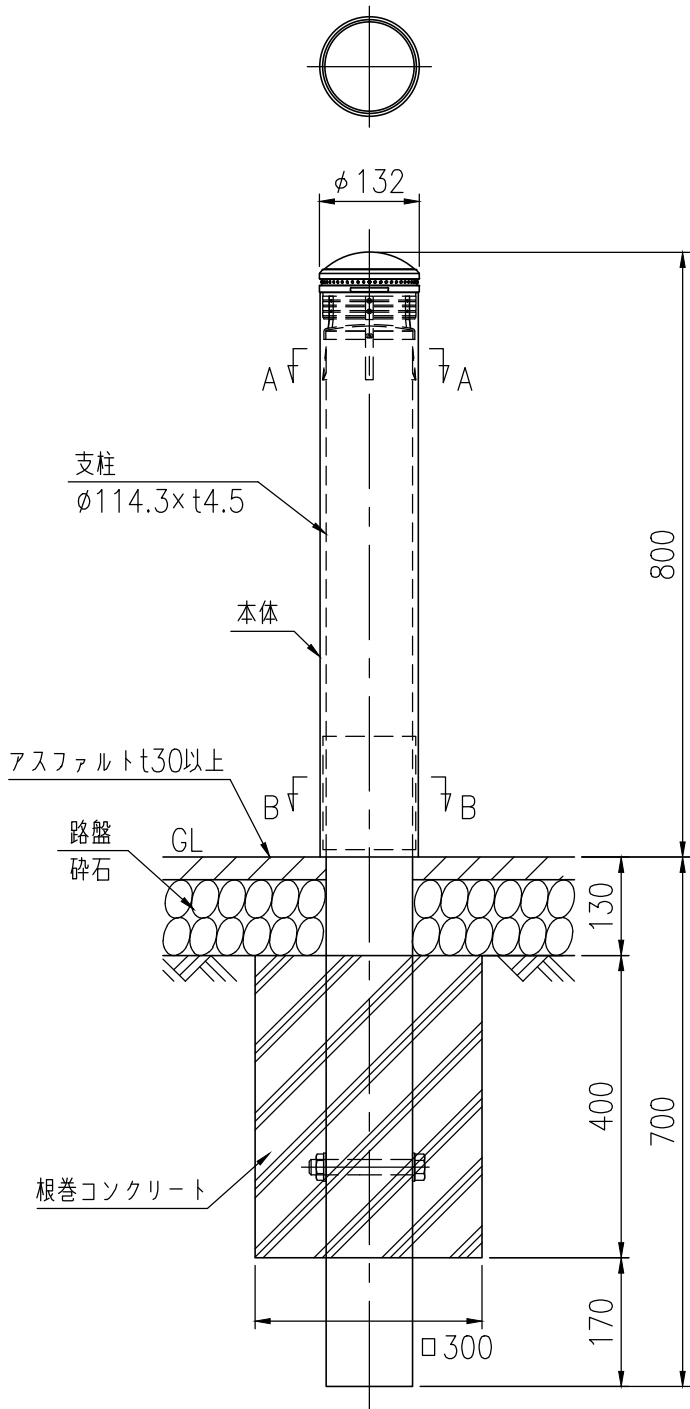
KDK-8SE (1/10)
