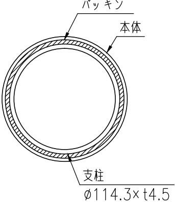
B-B 断面図 (1/4)
