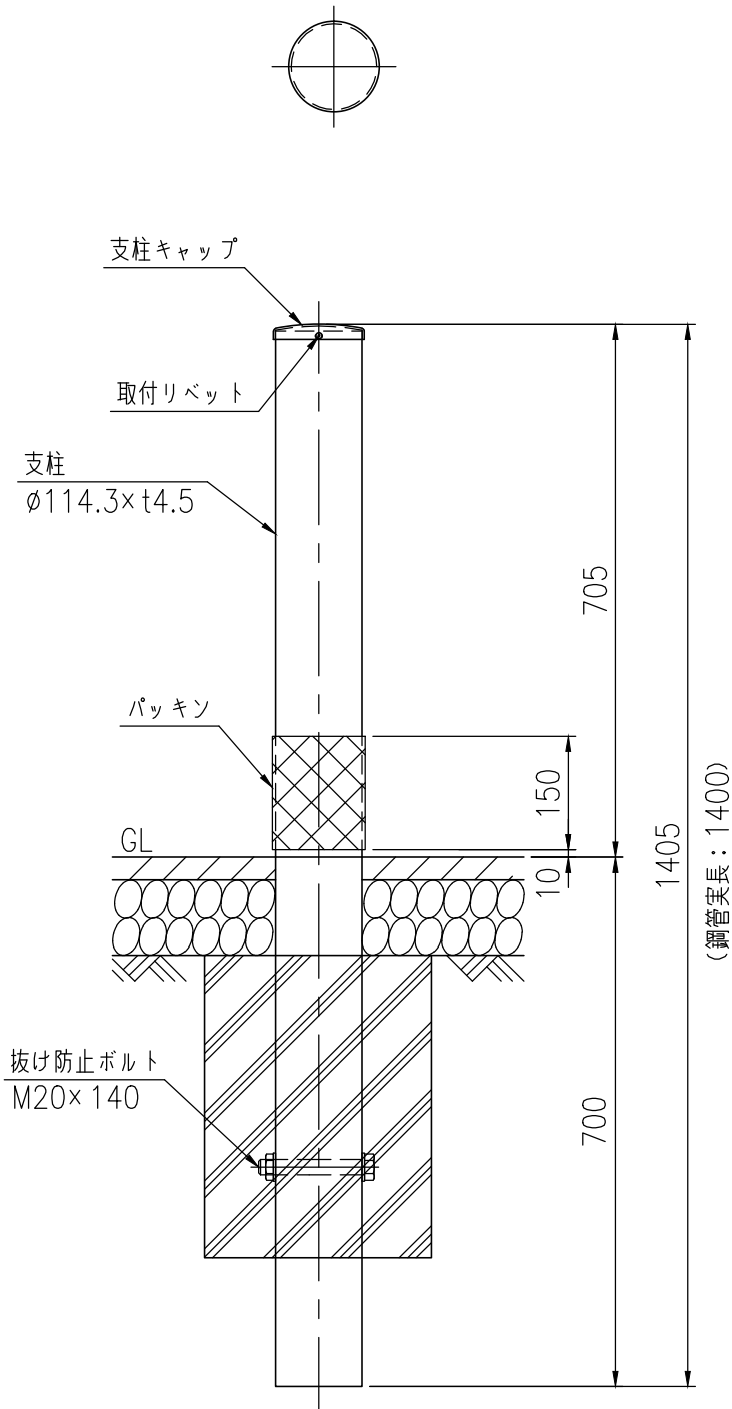
支柱姿図 (1/10)
