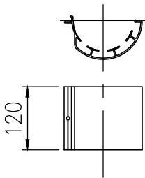
取付金具(1/10)
