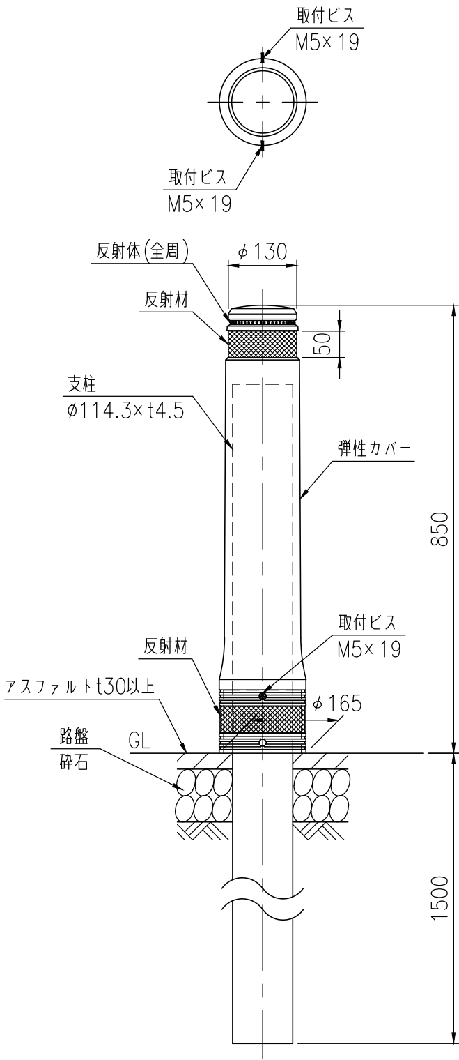
KDK-11E(1/10)
