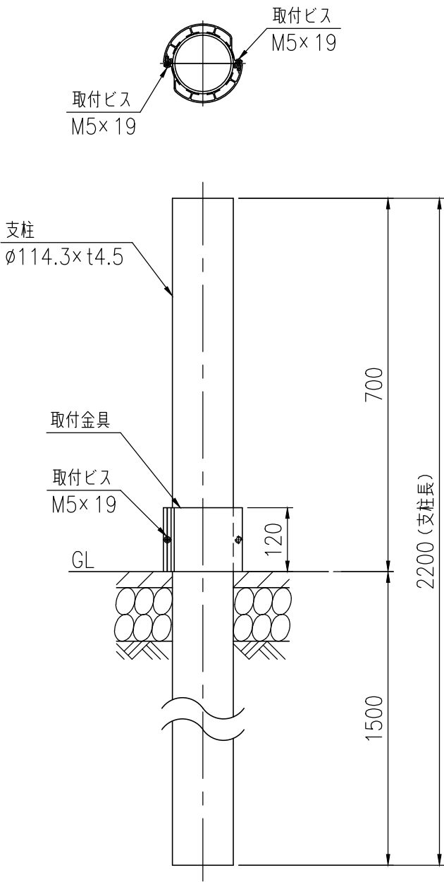
支柱設置図(1/10)
