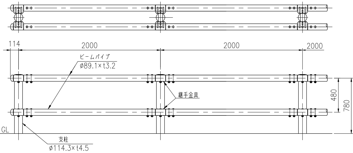
設置図 (1/25)
