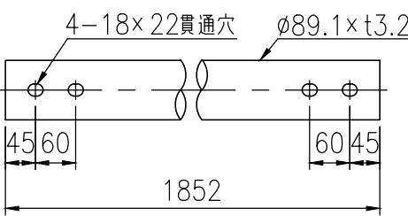
ビームパイプ詳細図 (1/10)
