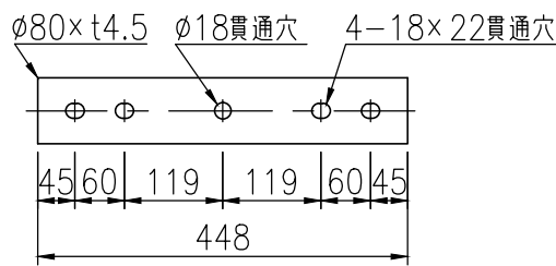
インナースリーブ詳細図 (1/10)
