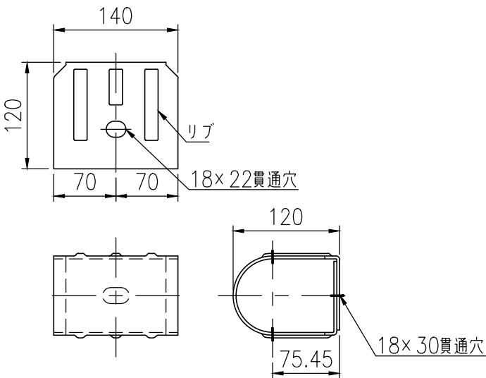
継手金具詳細図 (1/6)
