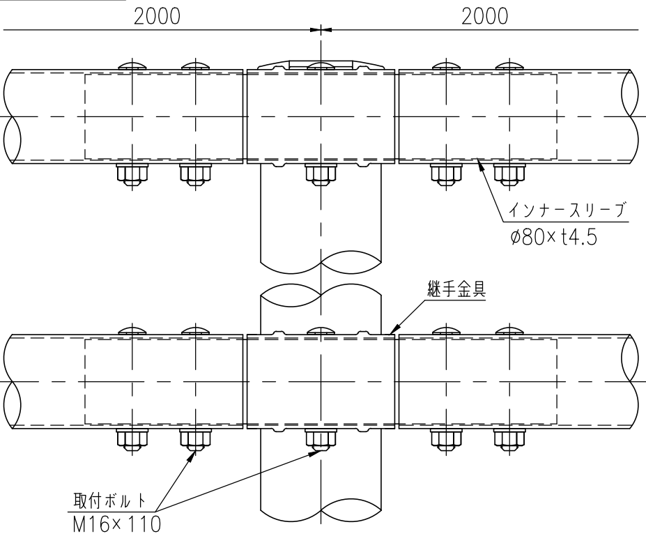
継手部詳細図 (1/5)
