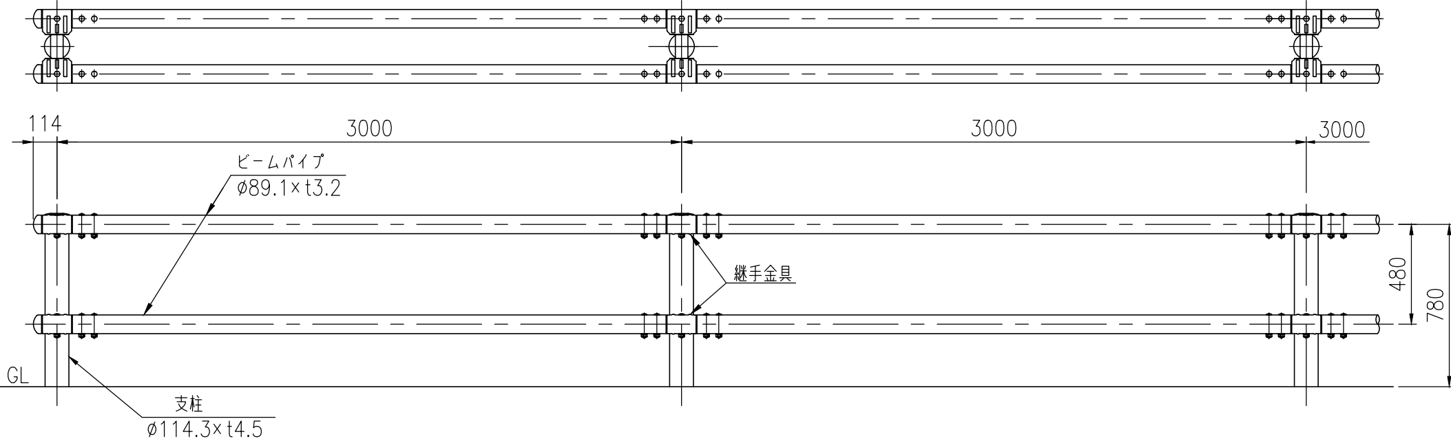
イソナー入リーブ詳細図 (1/10)
