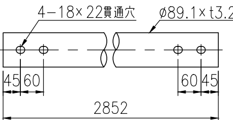
ビームパイプ詳細図 (1/10)
