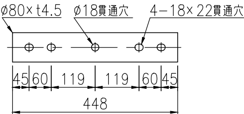
イソナー入リーブ詳細図 (1/10)
