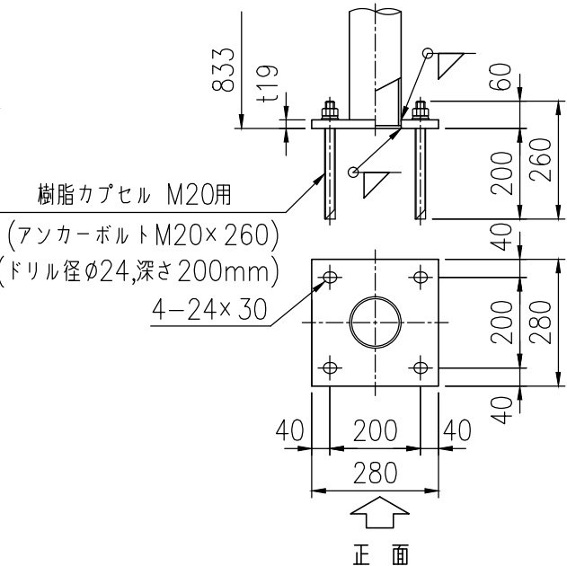
継手金具詳細図 (1/6)
