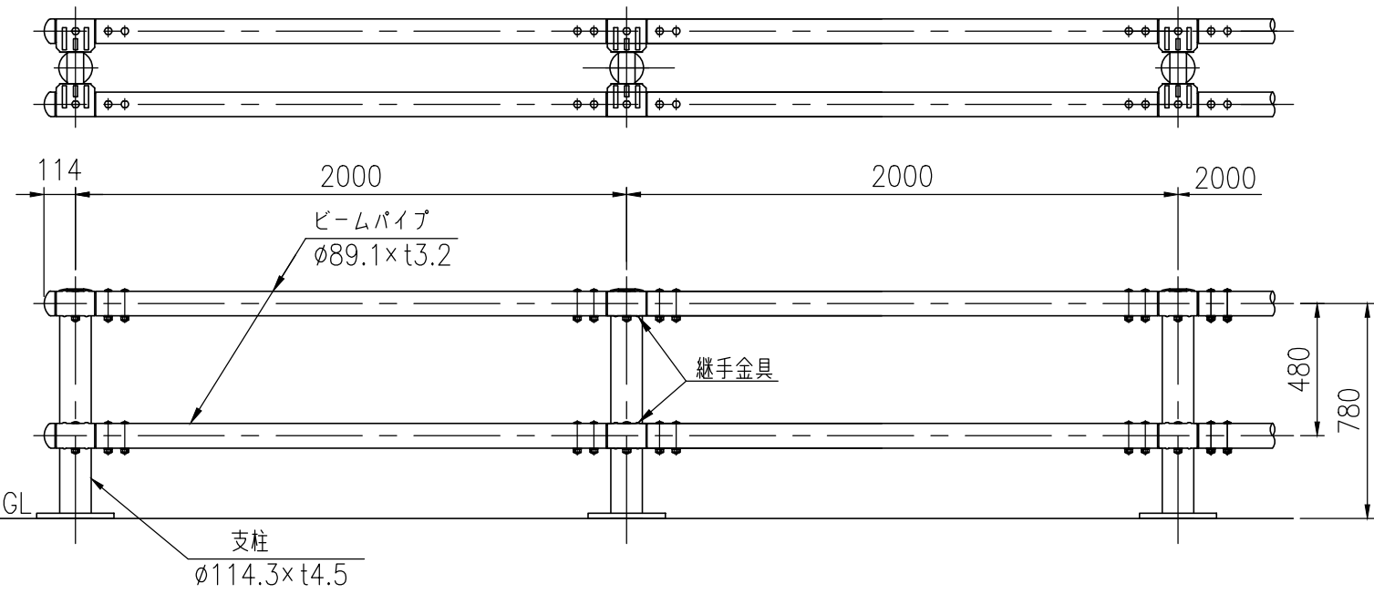
設置図 (1/25)
