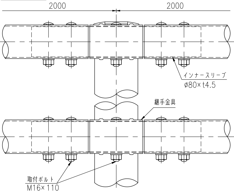
継手部詳細図 (1/5)
