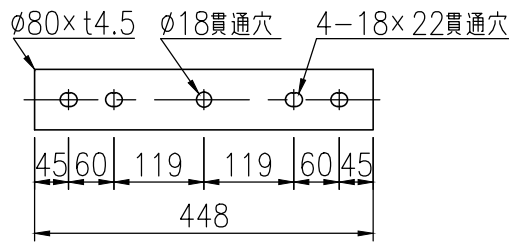
インナースリーブ詳細図 (1/10)
