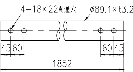
ビームパイプ詳細図 (1/10)
