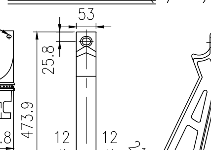
手摺受け金具詳細図 (1/10)
