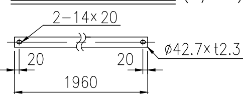
下段ビームパイプ詳細図 (1/16)
