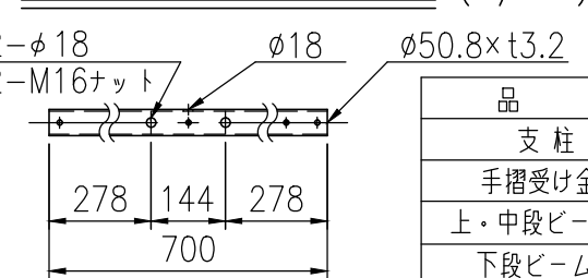
手摺インナースリーブ詳細図 (1/16)
