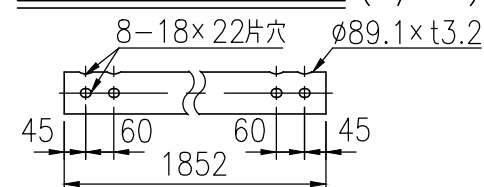
上段ビームパイプ詳細図 (1/16)
