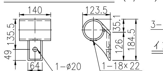
上段ビームコネクター詳細図 (1/10)
