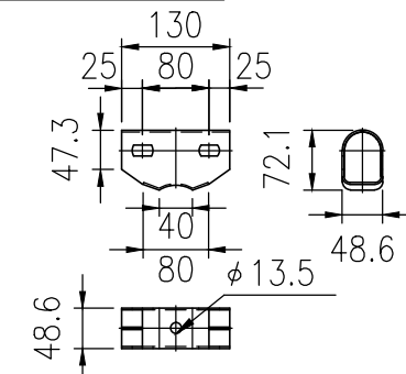
下段ビーム継手金具詳細図 (1/10)
