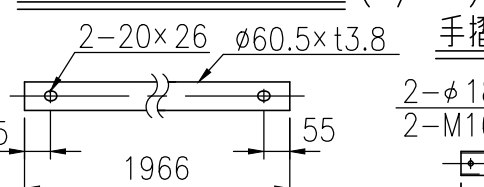
手摺ビームパイプ詳細図 (1/16)
