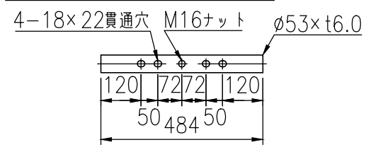
中段インナースリーブ詳細図 (1/16)
