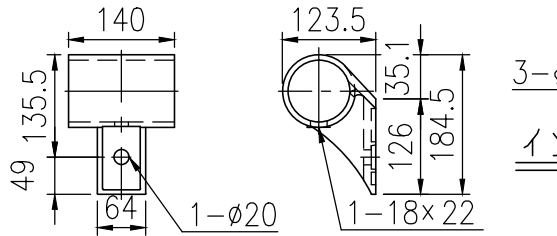
継手詳細図 (1/8)
