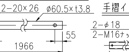
手摺ビームパイプ詳細図 (1/16)
