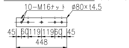
中段インナースリーブ詳細図 (1/16)
