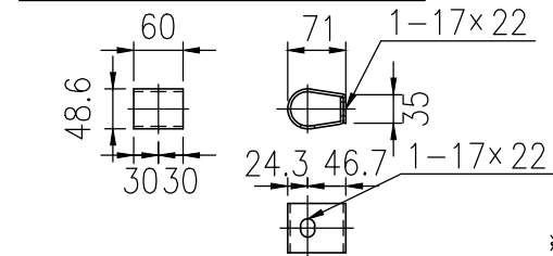
手摺インナースリーブ詳細図 (1/16)
