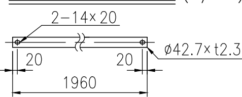
中段ビーム継手金具詳細図 (1/10)
