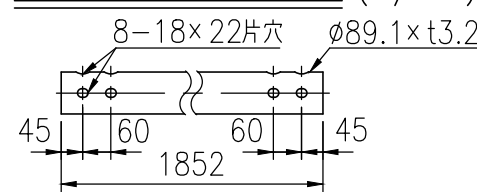
中段ビームパイプ詳細図 (1/16)
