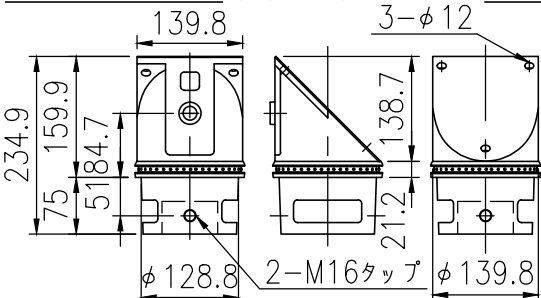
上段ビームコネクター詳細図 (1/10)
