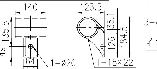
継手詳細図 (1/8)
