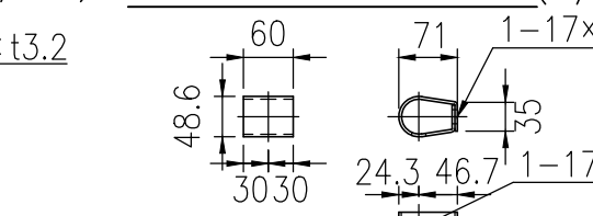
手摺インナー Sleeve 詳細図 (1/16)
