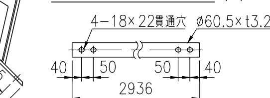
手摺ビームパイプ詳細図 (1/16)
