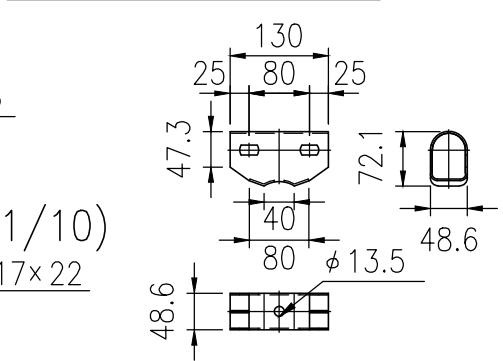
下段ビーム継手金具詳細図 (1/10)
