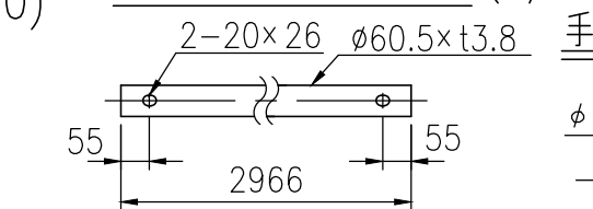
手摺ビームパイプ詳細図 (1/16)
