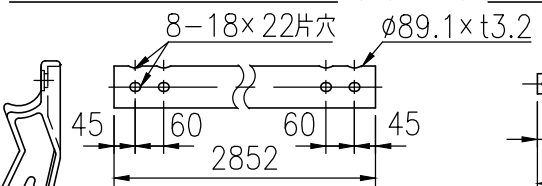
中段ビームパイプ詳細図 (1/16)
