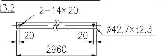
中段ビーム継手金具詳細図 (1/10)
