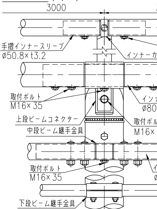
継手詳細図 (1/8)
