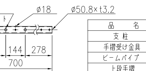
上段インナー Sleeve 詳細図 (1/16)
