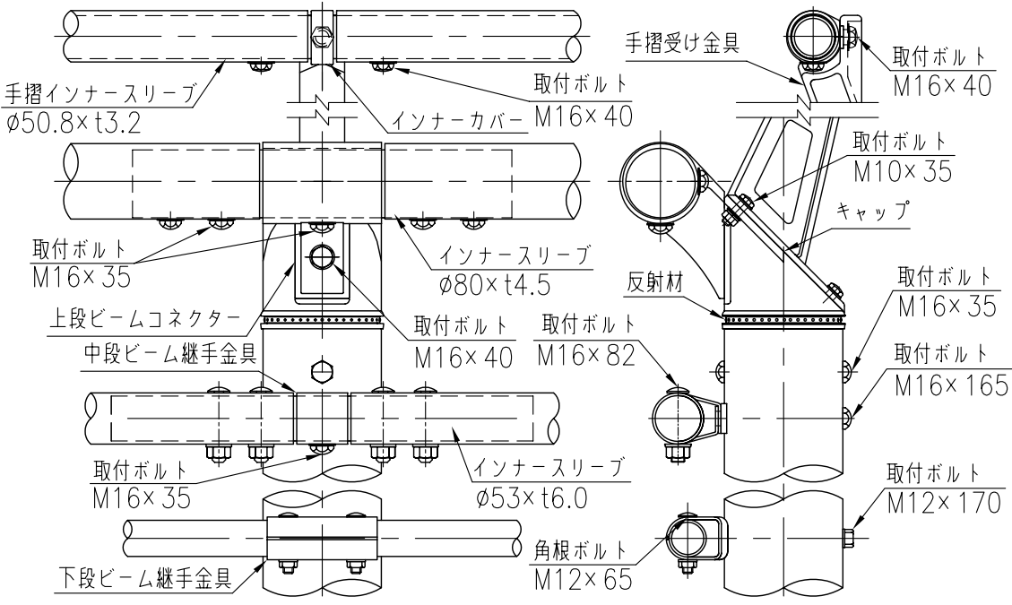
継手詳細図 (1/8)
