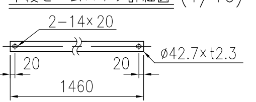
中段パイプ継手金具詳細図 (1/10)
