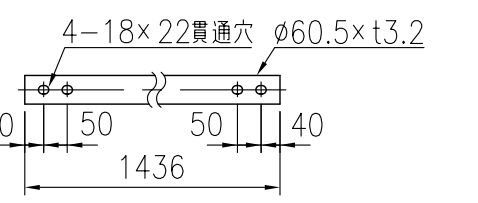
手摺パイプ詳細図 (1/16)
