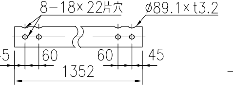
中段パイプ詳細図 (1/16)
