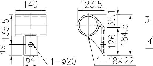
継手詳細図 (1/8)
