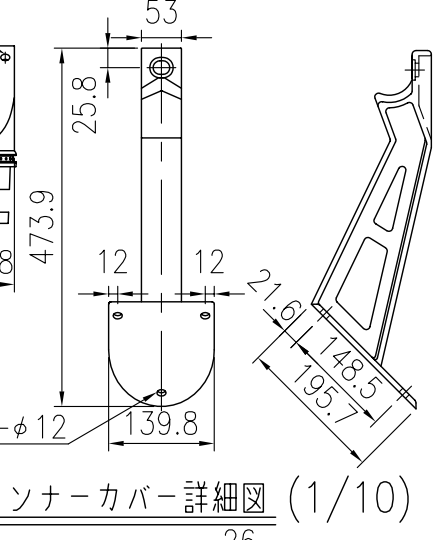
手摺受け金具詳細図 (1/10)
