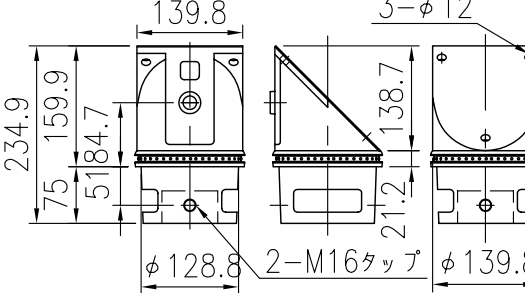
上段パイプコネクター詳細図 (1/10)
