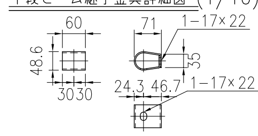
手摺インナー Sleeve 詳細図 (1/16)
