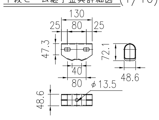
下段パイプ継手金具詳細図 (1/10)
