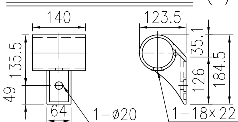
継手詳細図 (1/8)
