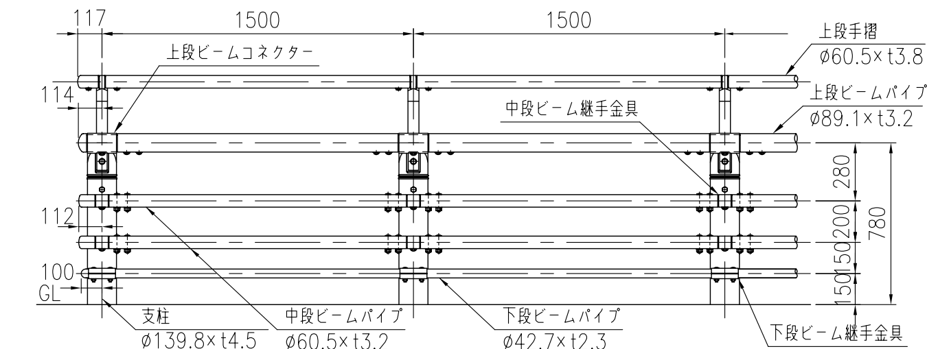
キャップ詳細図 (1/10)
