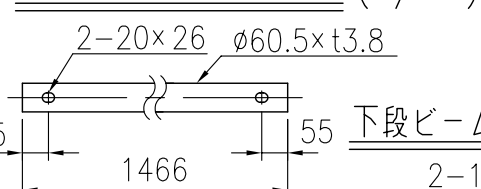
手摺ビームパイプ詳細図 (1/16)
