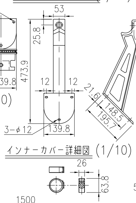
手摺受け金具詳細図 (1/10)
