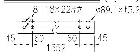
中段ビームパイプ詳細図 (1/16)
