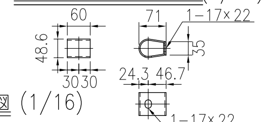
中段ビーム継手金具詳細図 (1/10)
