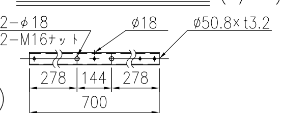
手摺インナースリーブ詳細図 (1/16)
