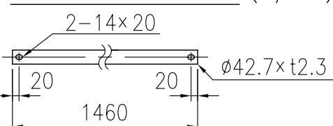
上段インナースリーブ詳細図 (1/16)
