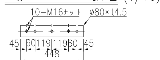
中段インナースリーブ詳細図 (1/16)
