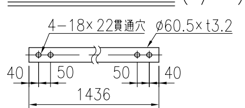
手摺ビームパイプ詳細図 (1/16)
