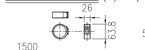
インナーカバー詳細図 (1/10)
