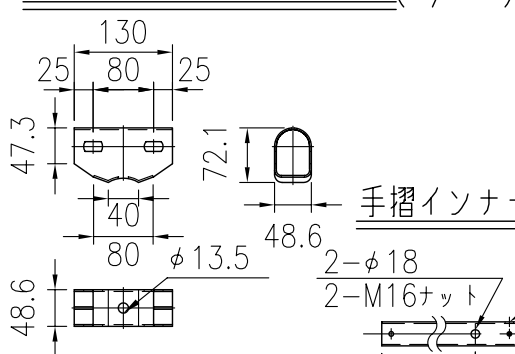
下段ビームパイプ詳細図 (1/16)
