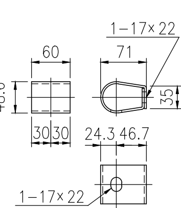
下段ビーム継手金具詳細図 (1/6)
