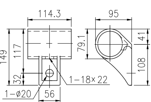
上段ビームコネクター詳細図 (1/6)
