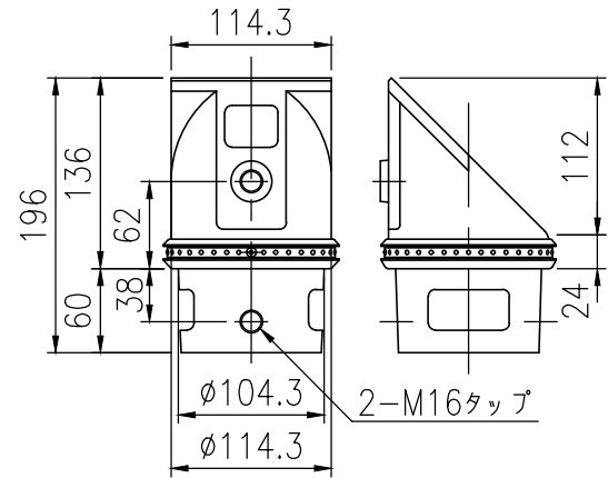
キャップ詳細図 (1/6)
