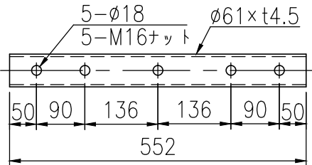
上段インナースリーブ詳細図 (1/10)
